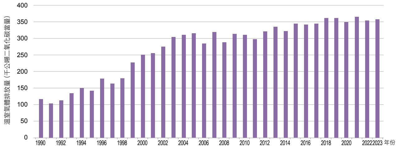
圖 4.3.9 1990 年至 2023 年氯乙烯生產製程排放量趨勢
