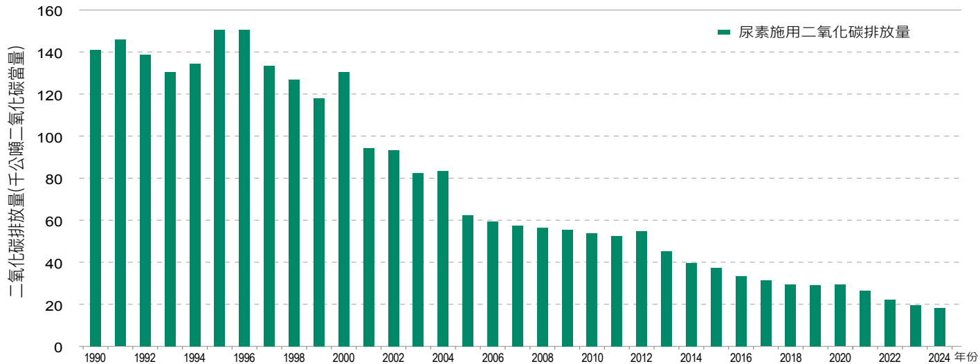
圖 5.9.1 1990 年至 2024 年尿素施用二氧化碳排放趨勢
