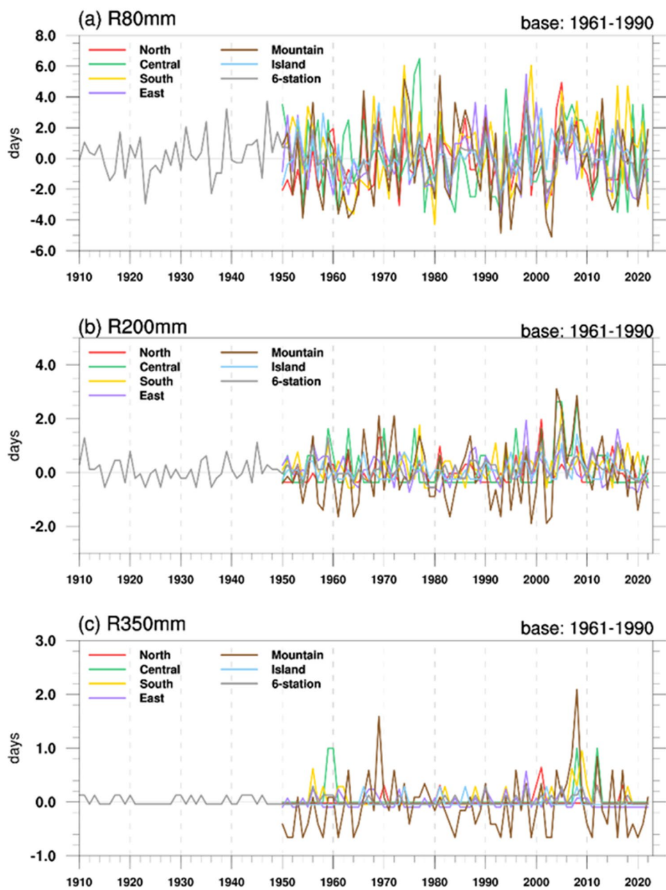
圖 5.1.4- 4 自 1910 年至 2021 年每年雨量超過 ( a ) 大雨門檻 80 毫米、( b ) 豪雨門檻 200 毫米及 ( c ) 大豪雨門檻 350 毫米總日數之距平時序圖。各測站氣候值為 1961 年至 1990 年之平均。線條顏色分別代表北部 ( 紅色 )、中部 ( 綠色 )、南部 ( 黃色 )、東部 ( 紫色 )、山區 ( 咖啡色 )、外島 ( 淺藍色 ) 及 6 個百年測站 ( 灰色 )。
