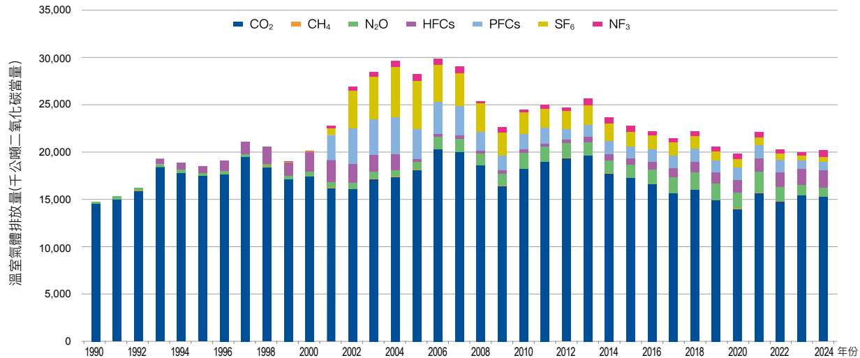
圖 4.1.4 1990 年至 2024 年工業製程及產品使用部門排放量趨勢（依氣體）
