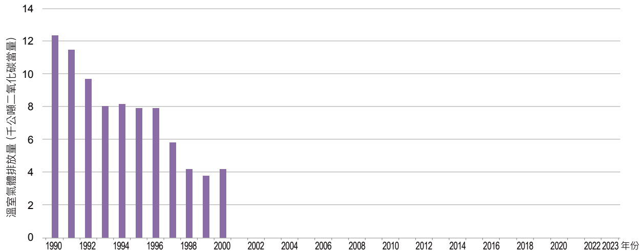
圖 4.3.6 1990 年至 2023 年純鹼生產製程排放量趨勢
