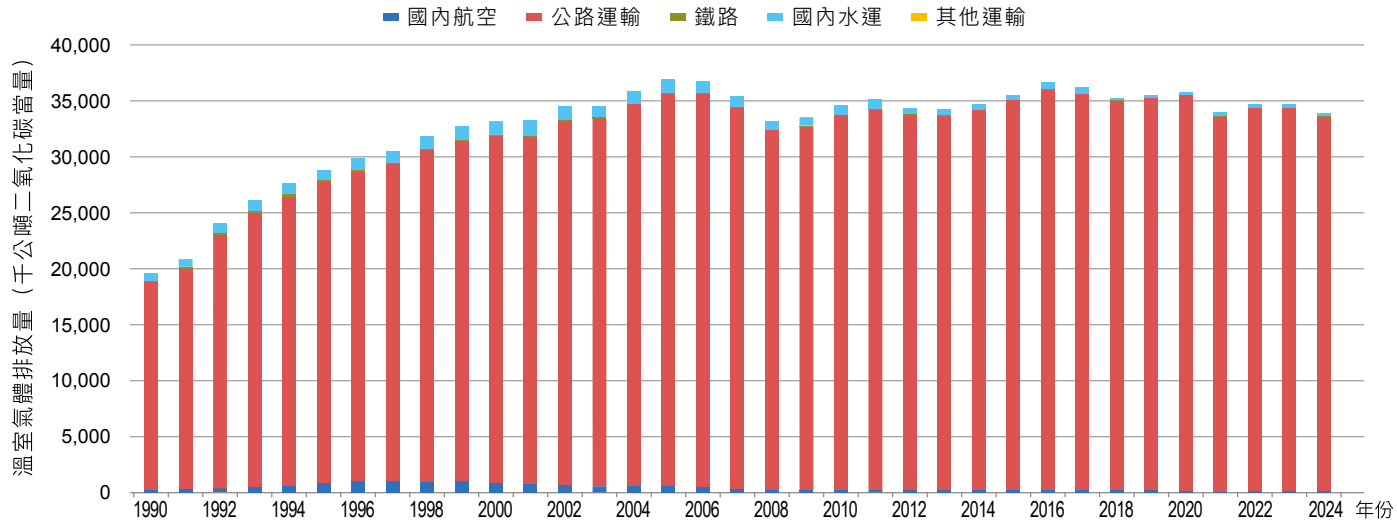
圖 3.2.29 1990 年至 2024 年運輸燃料燃燒二氧化碳排放量趨勢
