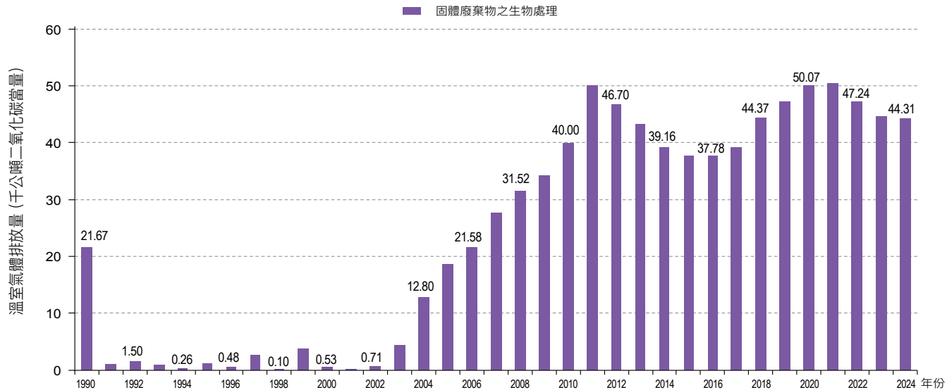
圖 7.3.1 1990 年至 2024 年固體廢棄物生物處理溫室氣體排放量趨勢
