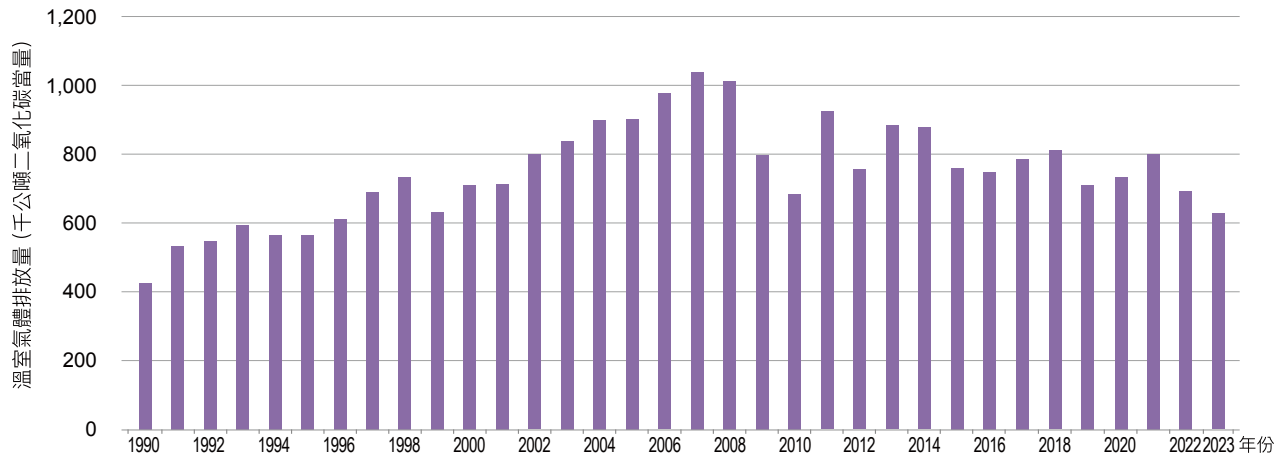
圖 4.4.3 1990 年至 2023 年電弧爐鋼胚生產製程排放量趨勢
