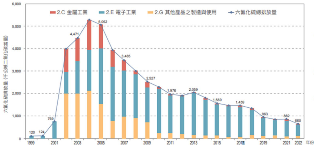
圖 2.3.6- 1 臺灣 1999 至 2022 年六氟化硫排放量趨勢
