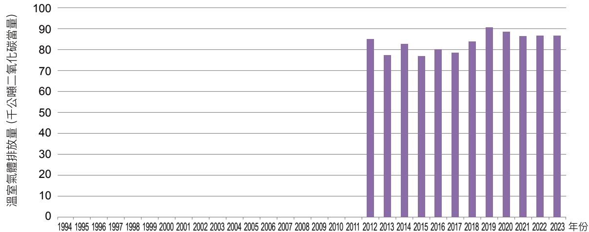
圖 4.7.2 1994 年至 2023 年家用冰箱之 HFCs 排放量趨勢
