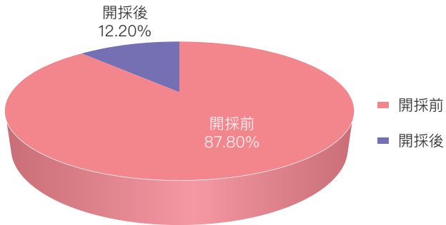
圖 3.3.4 2000 年固體燃料逸散溫室氣體排放占比
