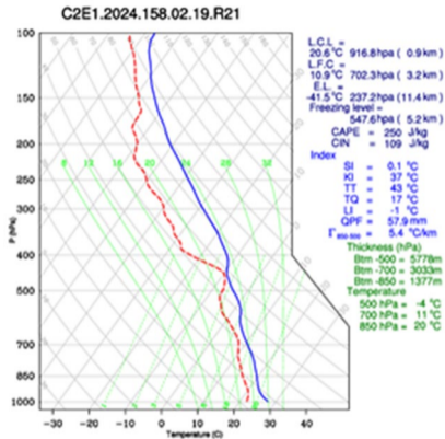
圖 6.2- 5 中央氣象署接收福衛七號所產製大氣垂直剖面（左）及全球溫度產品圖（右）
