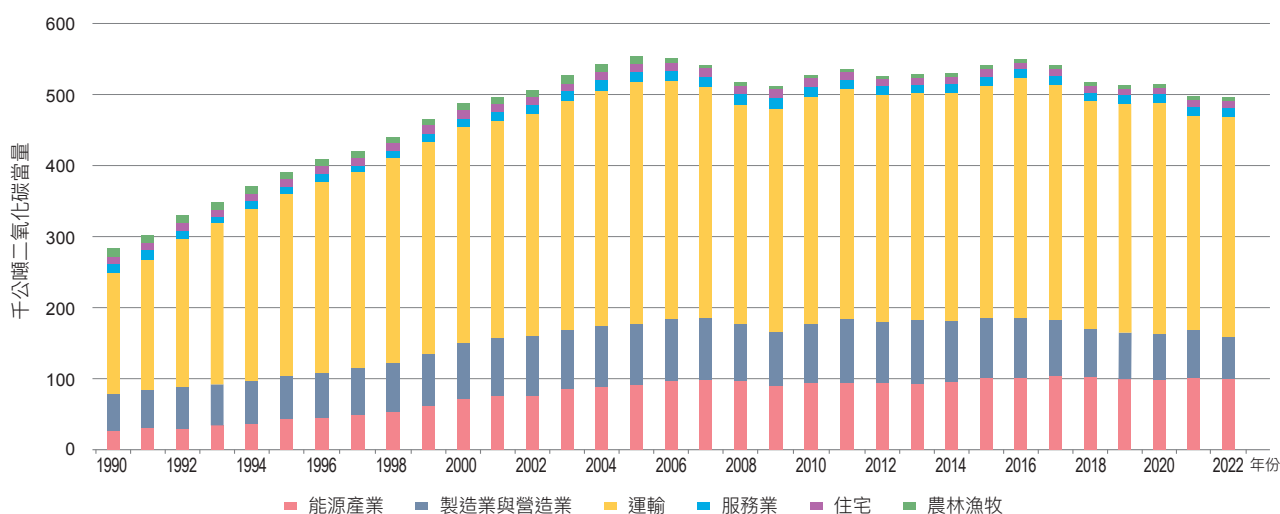
圖 3.2.3 1990 年至 2022 年能源部門燃料燃燒甲烷排放量趨勢
