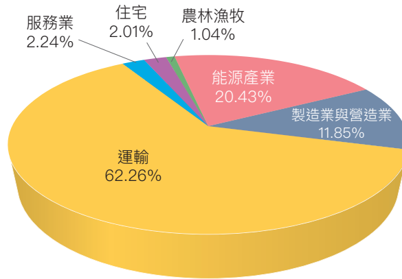
圖 3.2.4 2022 年能源部門燃料燃燒甲烷排放占比
