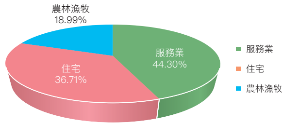
圖 3.2.29 2022 年服務業、住宅、農林漁牧燃料燃燒甲烷排放占比
