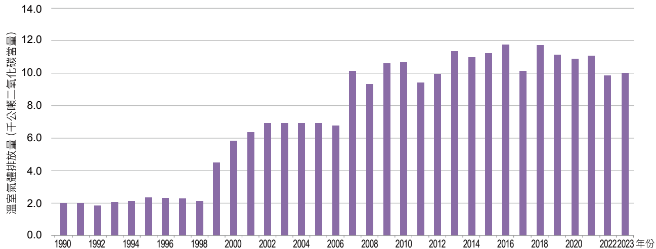
圖 4.3.14 1990 年至 2023 年苯乙烯生產製程排放量趨勢
