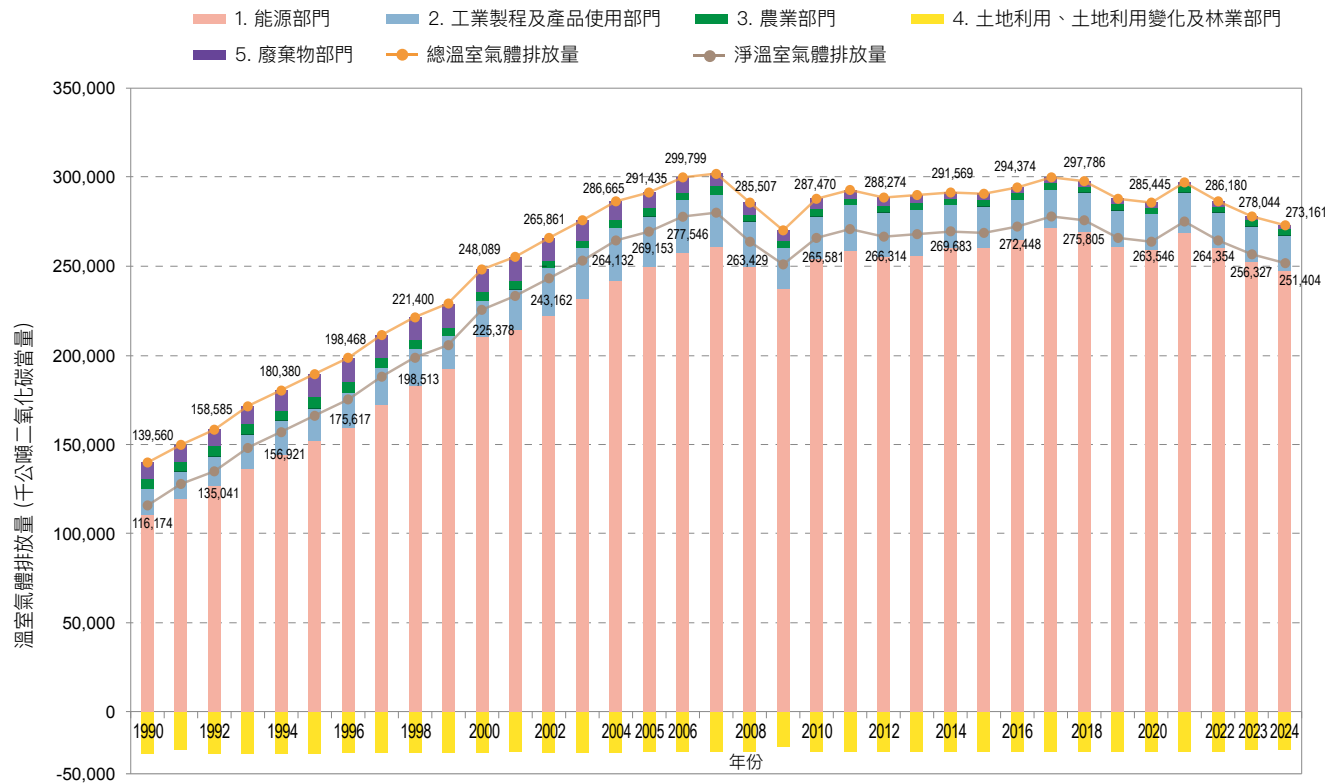
圖 2.3.1 1990 年至 2024 年各部門溫室氣體排放量趨勢
