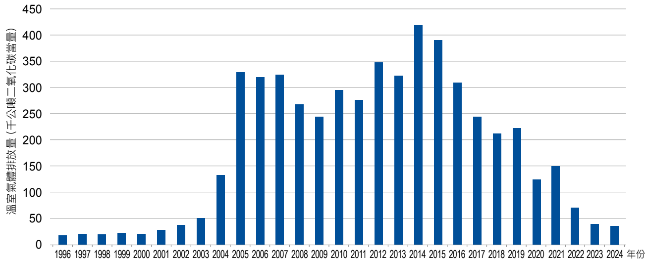
圖 4.3.10 1996 年至 2024 年環氧乙烷生產製程排放量趨勢
