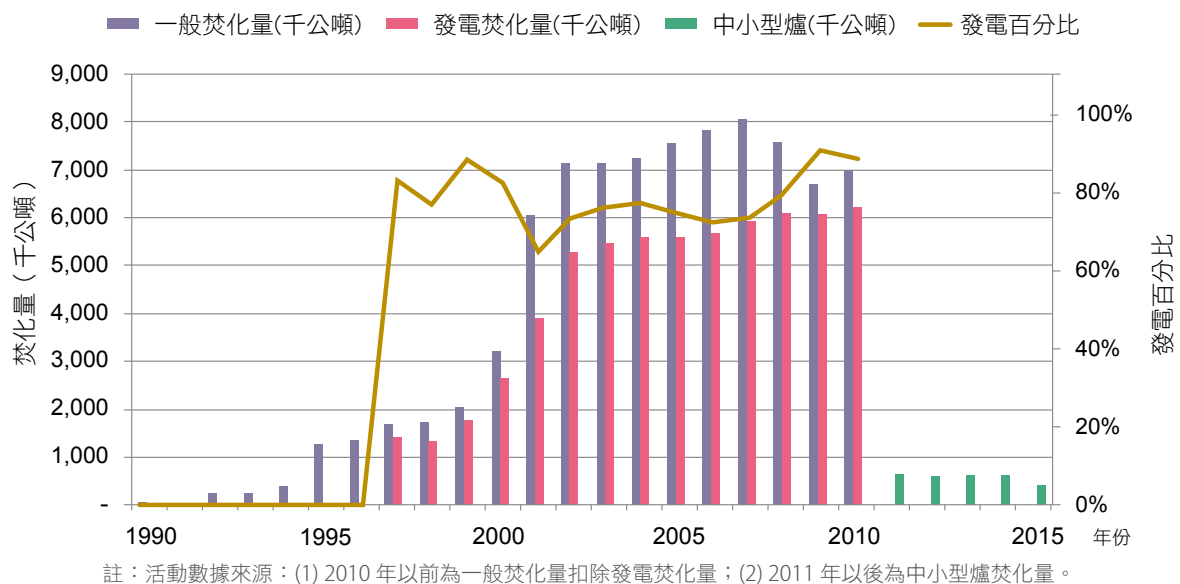
圖 7.4.1 臺灣 1990 至 2015 年發電焚化量近年變化趨勢
