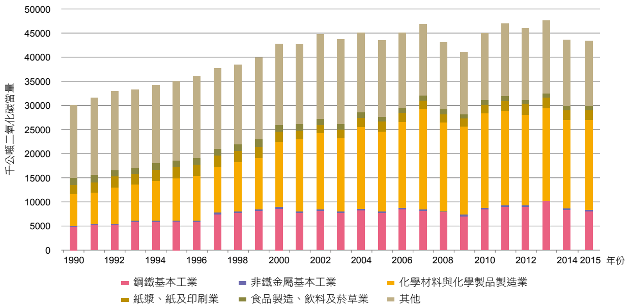
圖 3.2.14 臺灣 1990 至 2015 年製造業與營造業燃料燃燒二氧化碳排放趨勢
