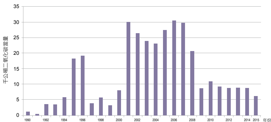
圖 7.4.3 臺灣 1990 至 2015 年廢棄物焚化氧化亞氮排放趨勢
