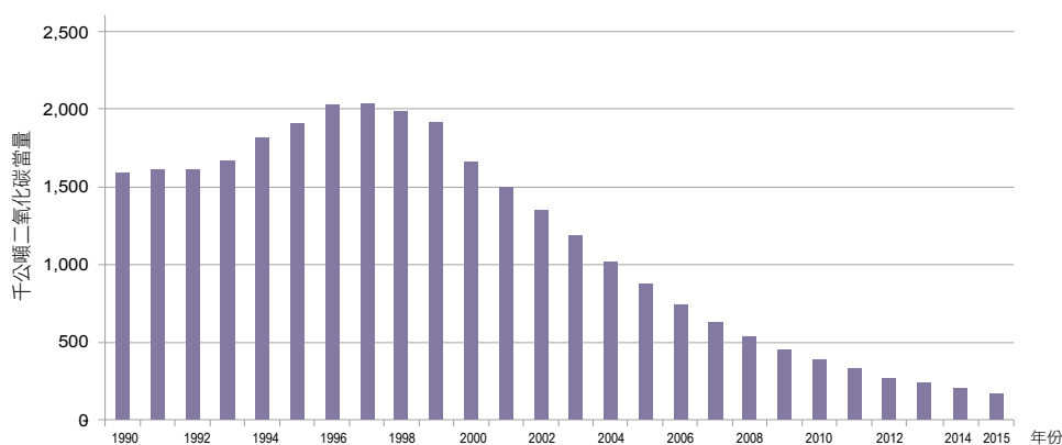
圖 7.2.2 臺灣 1990 至 2015 年未妥善管理廢棄物掩埋場甲烷排放量趨勢
