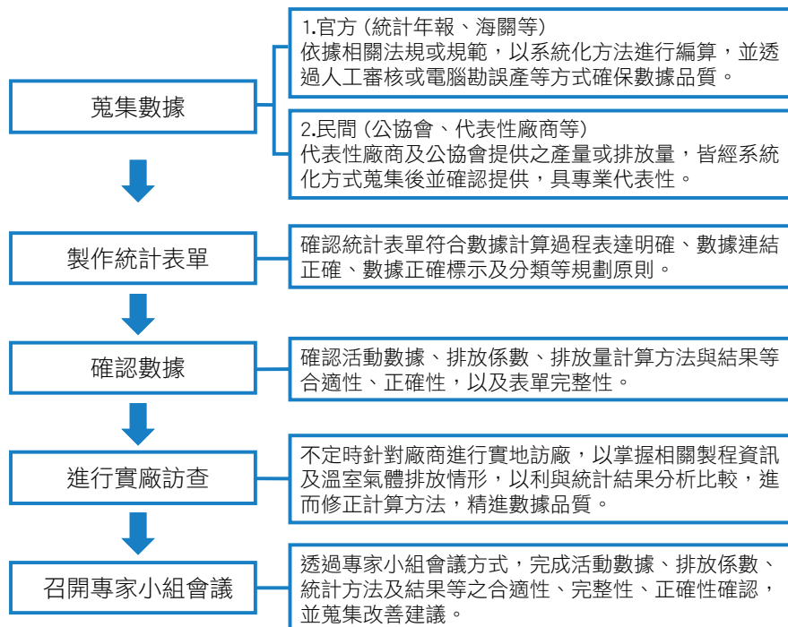
圖 4.3.3 工業製程及產品使用部門溫室氣體排放統計 QA/QC 流程（活動數據 - 官方數據、公協會及廠商來源）
