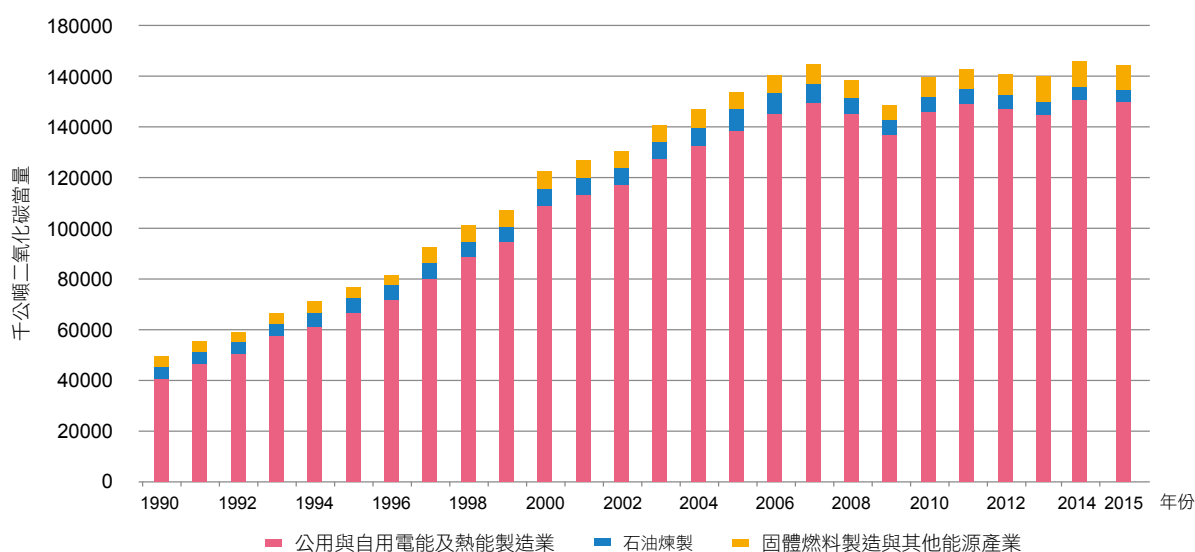
圖 3.2.8 臺灣 1990 至 2015 年能源產業燃料燃燒二氧化碳排放量趨勢
