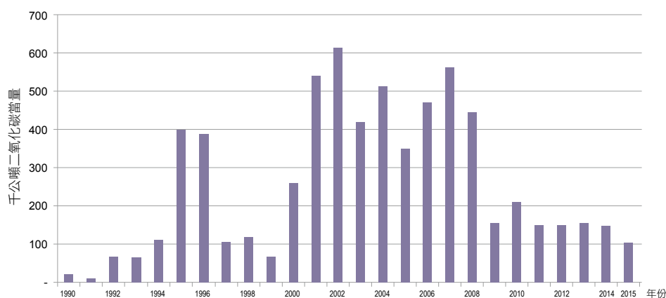
圖 7.4.2 臺灣 1990 至 2015 年廢棄物焚化二氧化碳排放量趨勢
