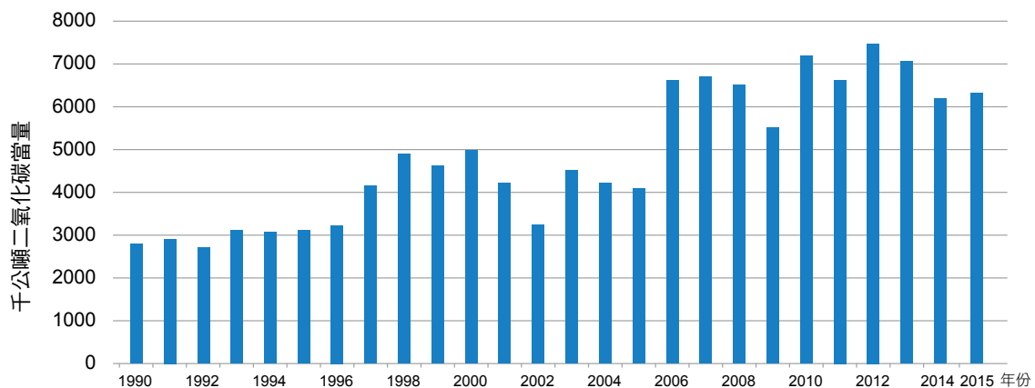
圖 4.4.2 臺灣 1990 至 2015 年高爐鋼胚生產排放量趨勢
