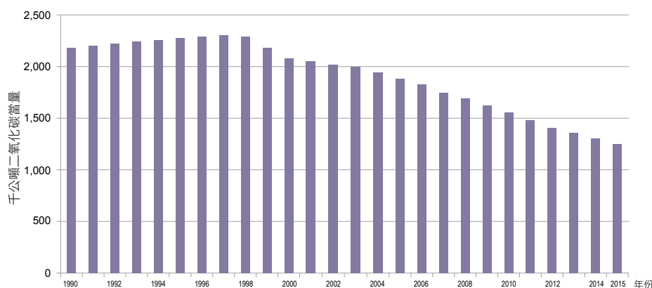
圖 7.5.1 臺灣 1990 至 2015 年全國生活污水處理甲烷排放趨勢
