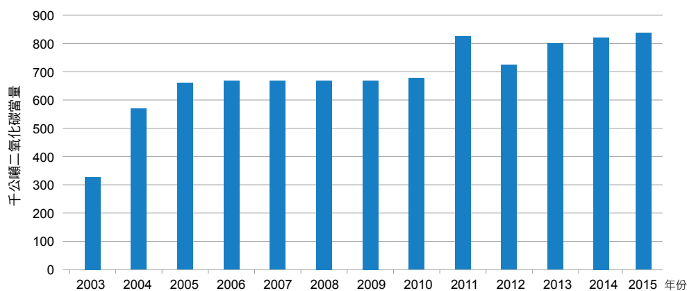
圖 4.7.2 臺灣 2003 至 2015 年冷凍空調使用排放量趨勢
