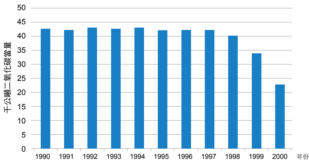
圖 4.3.5 臺灣 1990 至 2000 年碳化鈣使用排放量趨勢
