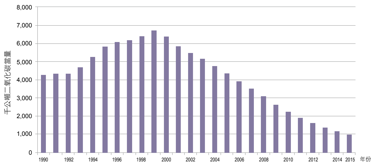
圖 7.2.1 臺灣 1990 至 2015 年衛生掩埋場甲烷排放量趨勢
