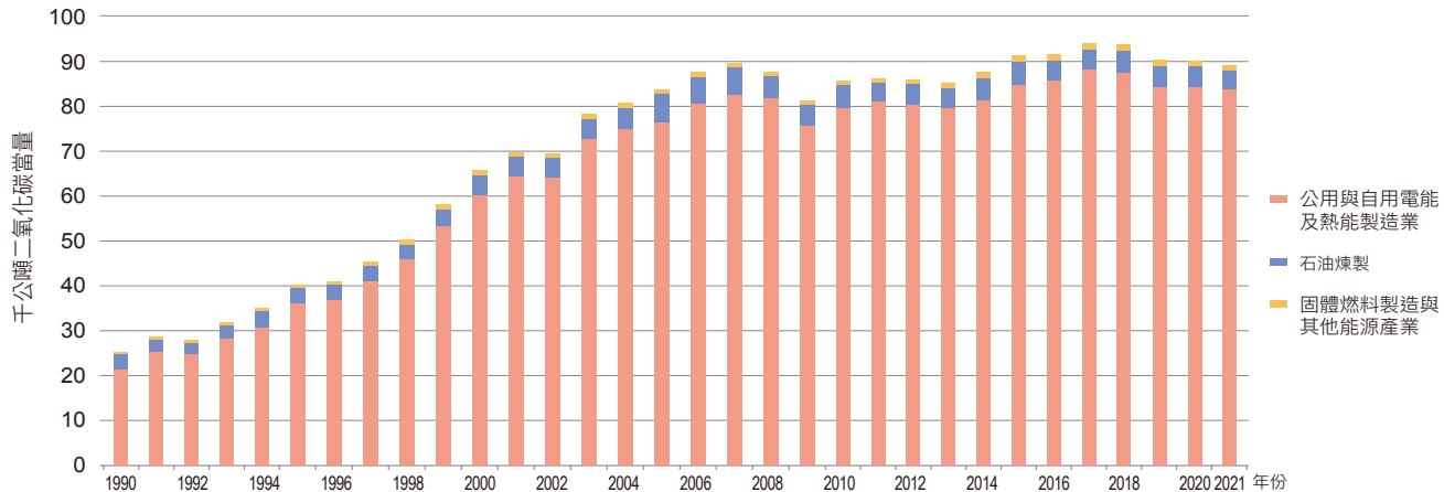
圖 3.2.10 1990 年至 2021 年能源產業燃料燃燒甲烷排放量趨勢
