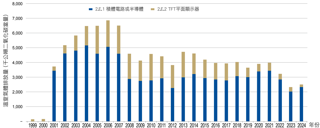
圖 4.6.1 1999 年至 2024 年電子工業製程排放量趨勢
