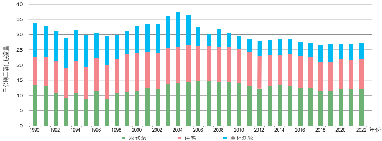
圖 3.2.28 1990 年至 2022 年服務業、住宅、農林漁牧燃料燃燒甲烷排放量趨勢
