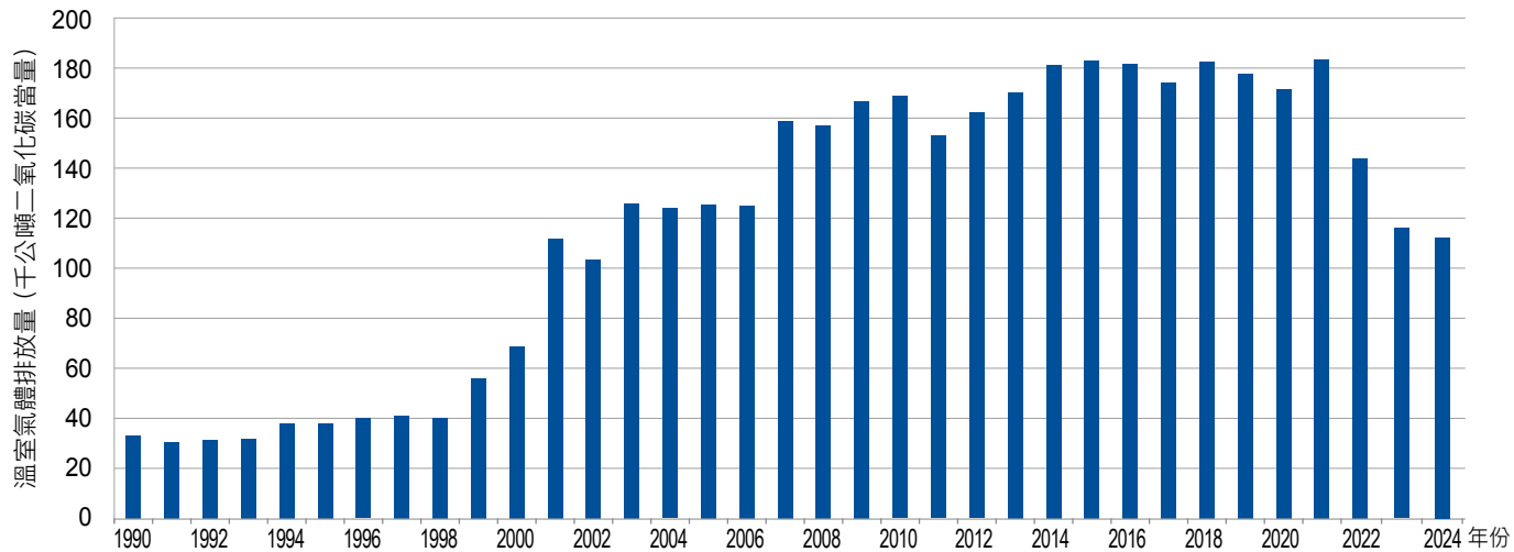
圖 4.3.8 1990 年至 2024 年乙烯生產製程排放量趨勢
