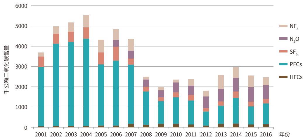
圖 4.6.2 臺灣 2001 至 2016 年積體電路或半導體排放量趨勢
