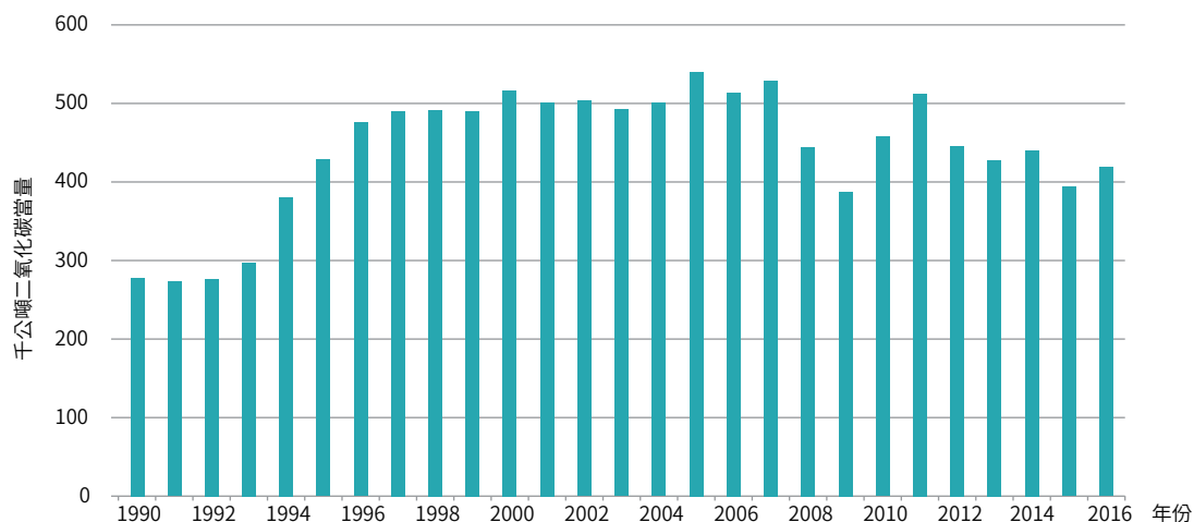
圖 4.3.13 臺灣 1990 至 2016 年碳黑生產排放量趨勢
