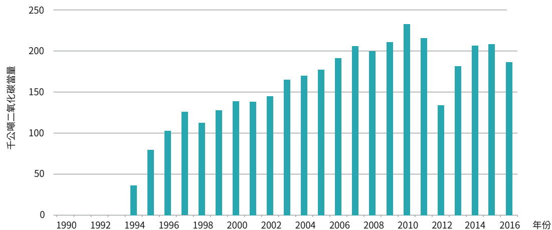
圖 4.3.6 臺灣 1990 至 2016 年二氧化鈦生產排放量趨勢
