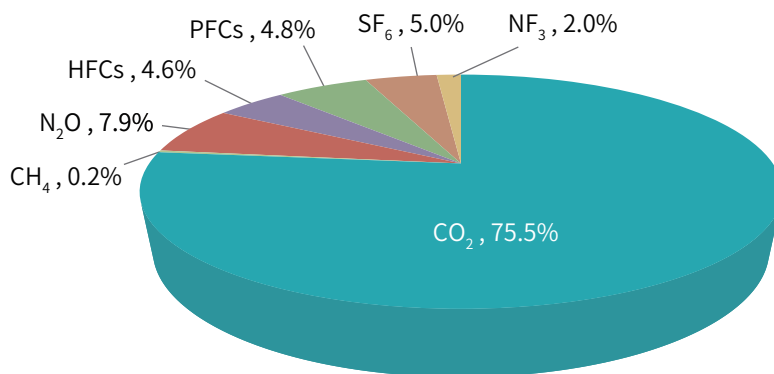
圖 4.1.1 臺灣 2016 年工業製程及產品使用部門溫室氣體種類排放占比
