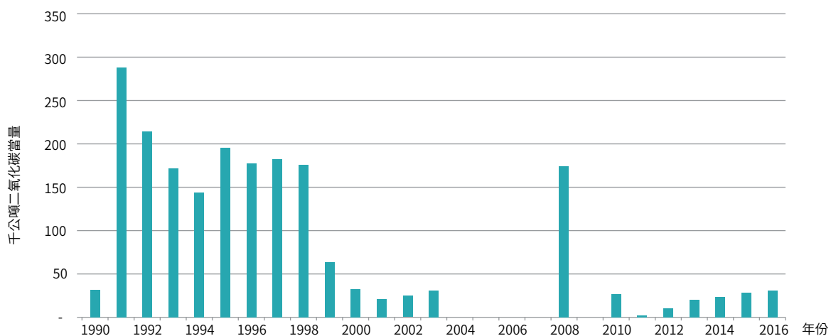
圖 4.4.4 臺灣 1990 至 2016 年鐵合金生產排放量趨勢
