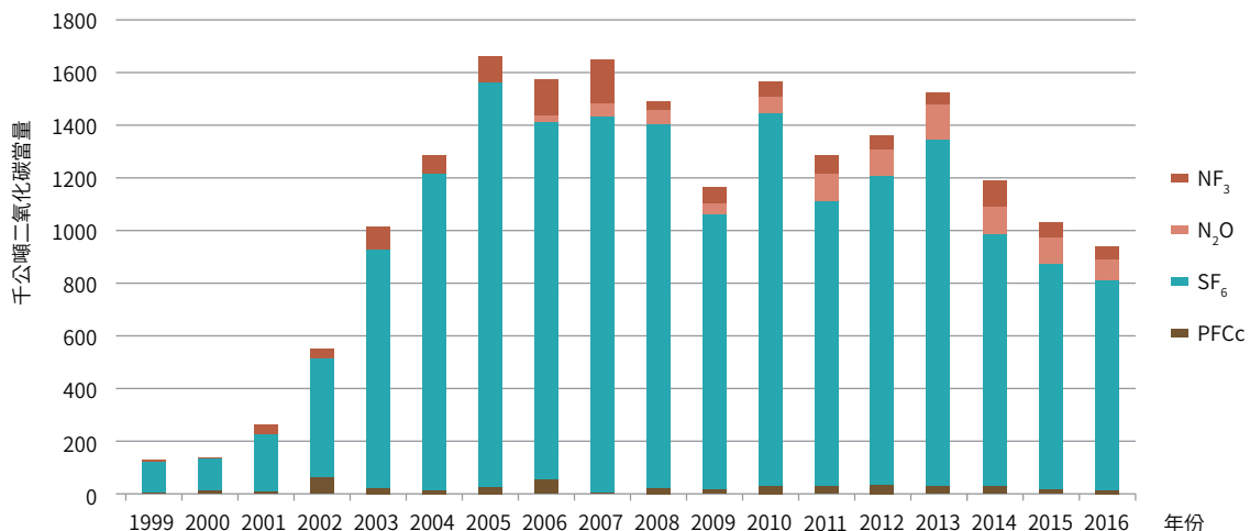
圖 4.6.4 臺灣 1999 至 2016 年 TFT 平面顯示器排放量趨勢
