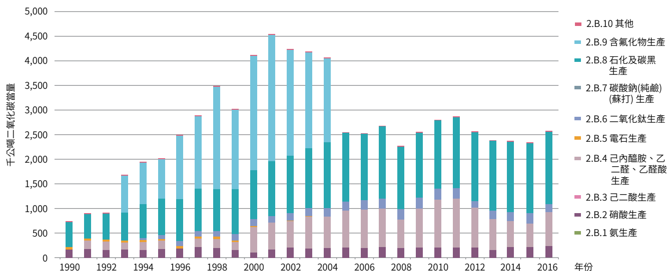
圖 4.3.1 臺灣 1990 至 2016 年化學工業排放量趨勢
