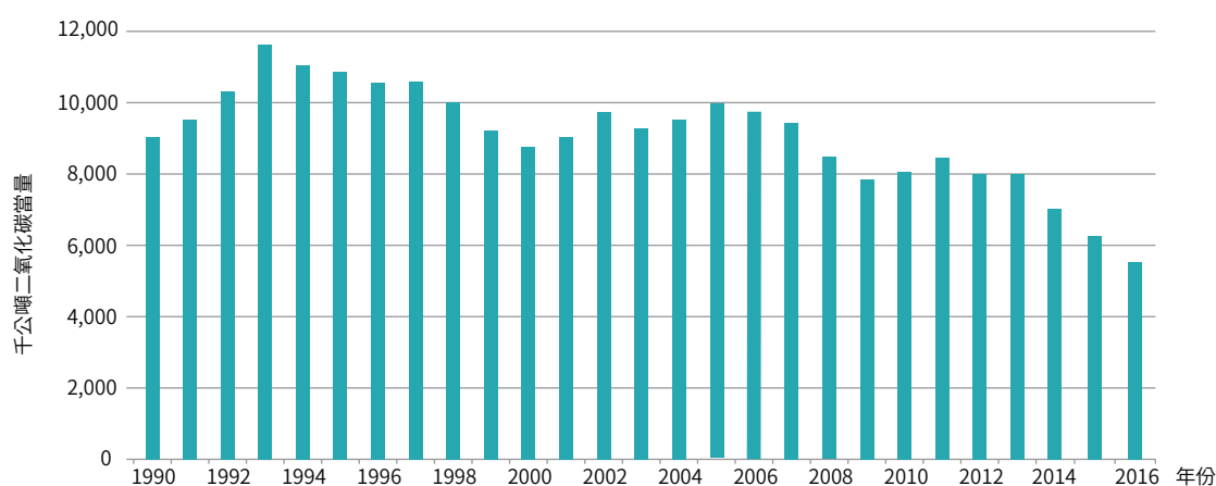
圖 4.2.2 臺灣 1990 至 2016 年水泥生產製程排放量趨勢
