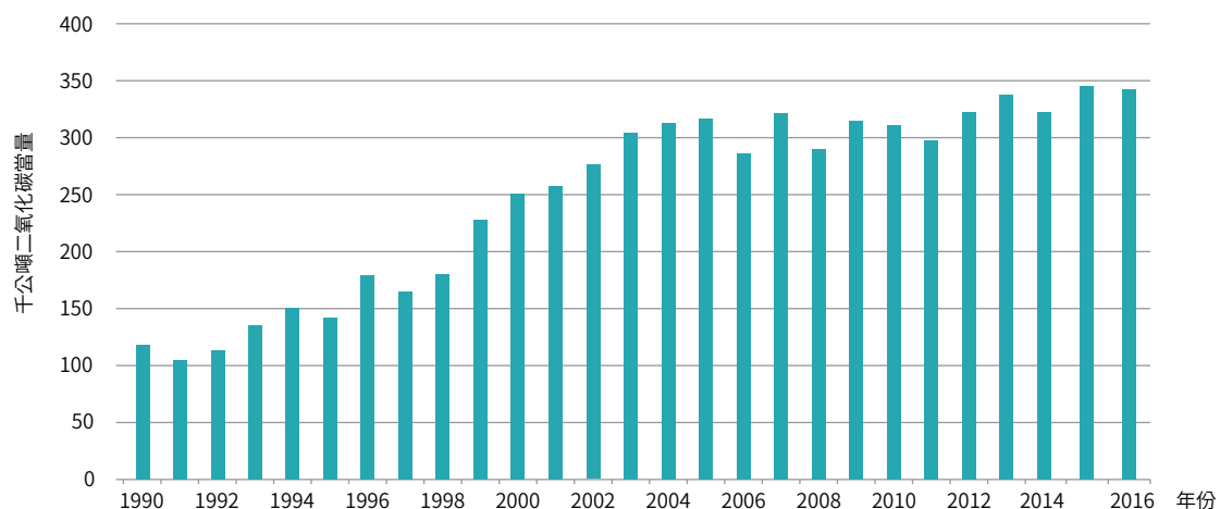
圖 4.3.10 臺灣 1990 至 2016 年氯乙烯生產排放量趨勢
