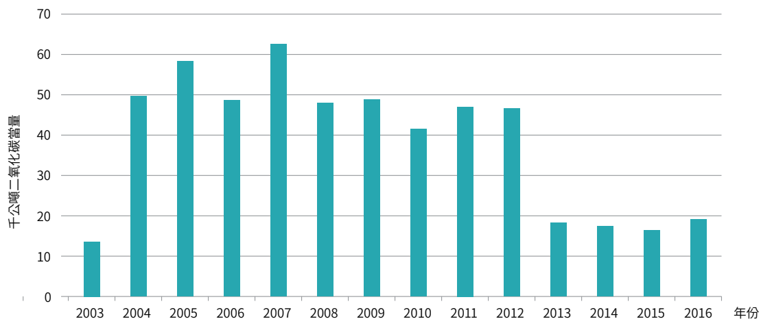
圖 4.4.8 臺灣 2003 至 2016 年鋅生產排放量趨勢
