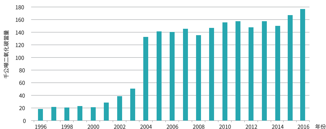
圖 4.3.11 臺灣 1996 至 2016 年環氧乙烷生產排放量趨勢
