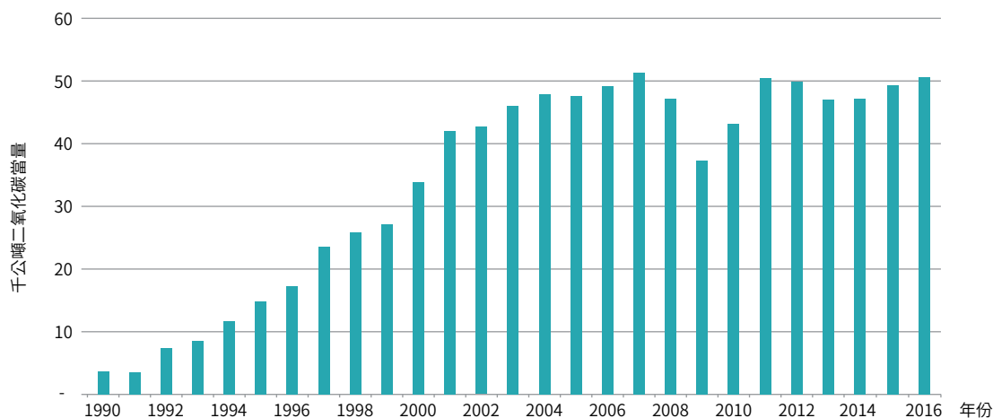
圖 4.2.9 臺灣 1990 至 2016 年玻璃纖維製品生產二氧化碳排放量趨勢
