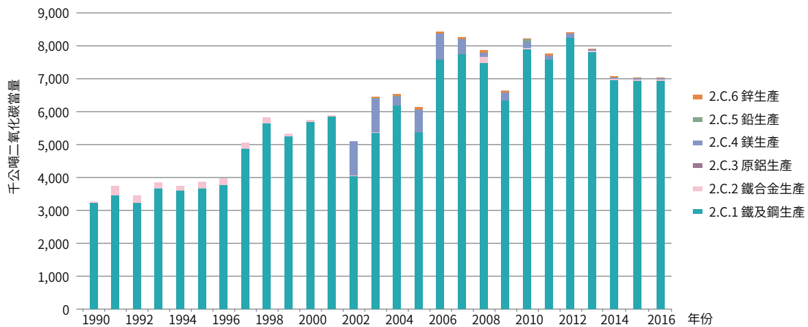
圖 4.4.1 臺灣 1990 至 2016 年金屬製程排放量趨勢
