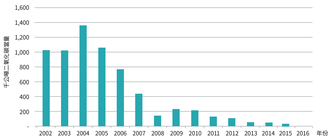
圖 4.4.5 臺灣 2002 至 2016 年鎂生產排放量趨勢
