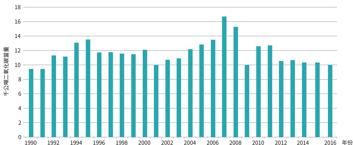
圖 4.2.6 臺灣 1990 至 2016 年玻璃生產排放量趨勢
