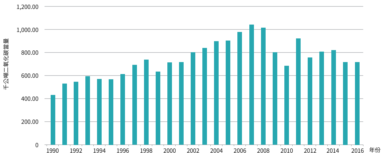
圖 4.4.3 臺灣 1990 至 2016 年電弧爐鋼胚生產排放量趨勢
