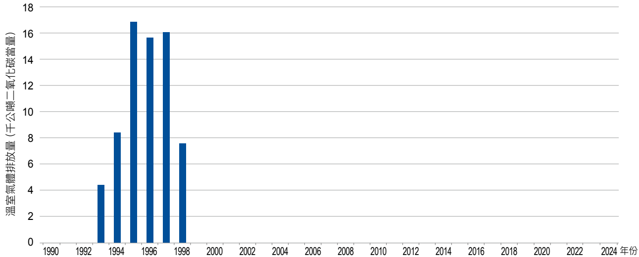
圖 4.3.7 1990 年至 2024 年甲醇生產製程排放量趨勢
