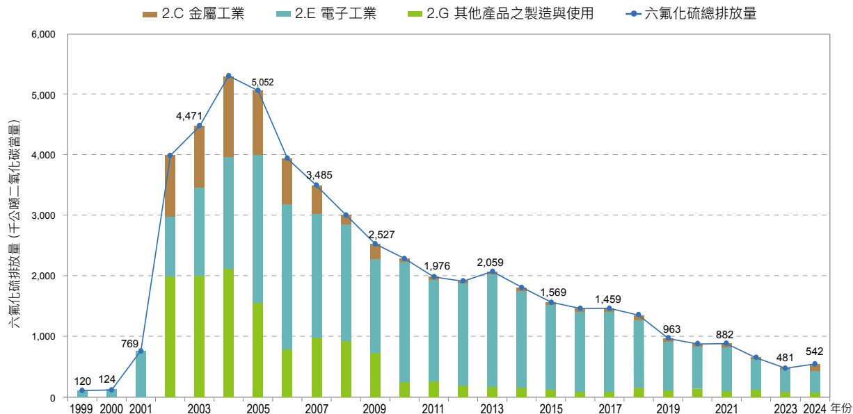
圖 2.2.6 1999 年至 2024 年六氟化硫排放量趨勢
