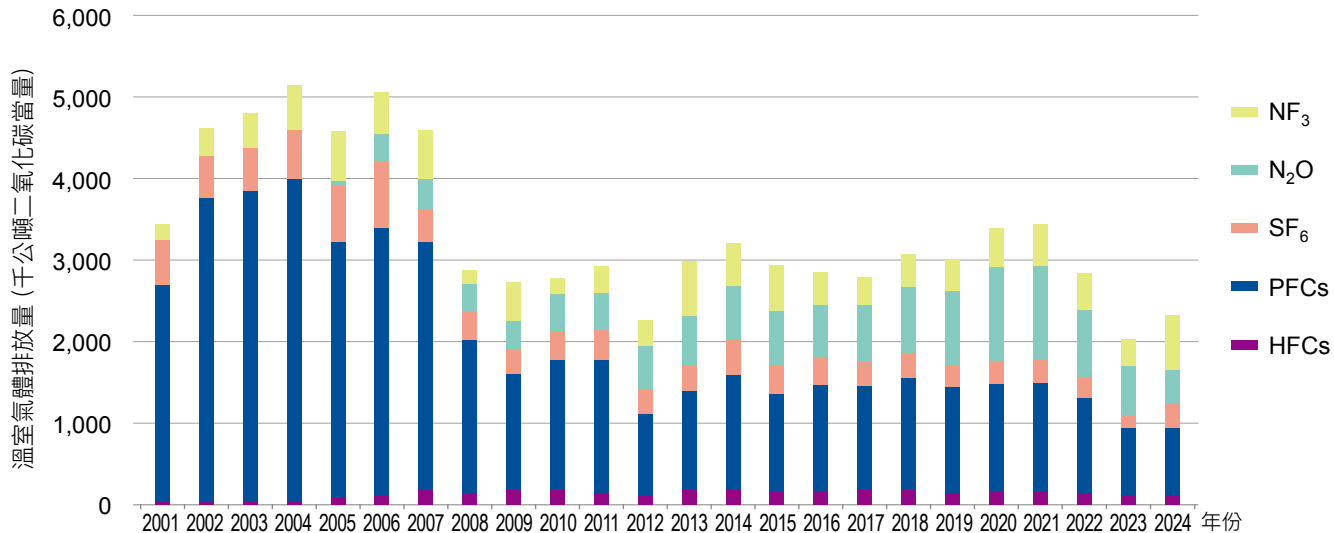
圖 4.6.2 2001 年至 2024 年積體電路及半導體製程排放量趨勢
