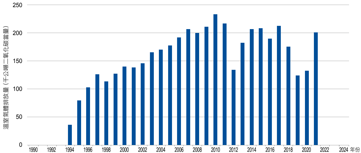
圖 4.3.5 1990 年至 2024 年二氧化鈦生產製程排放量趨勢
