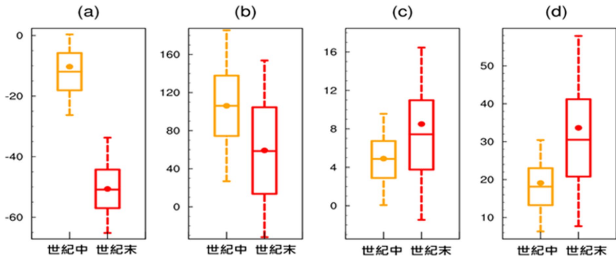
圖 5.1.4- 1 RCP8.5 情境下，21 世紀中（黃色）與世紀末（紅色）的（a）影響臺灣颱風頻率、（b）強颱風頻率、（c）近中心最大風速、（d）距中心 200km 內平均雨量的模擬結果
