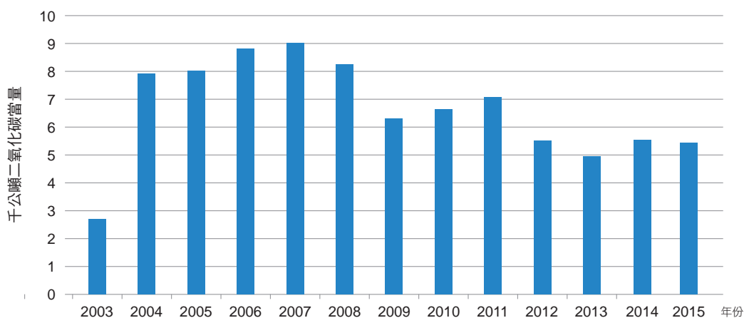
圖 4.4.7 臺灣 2003 至 2015 年鉛生產排放量趨勢
