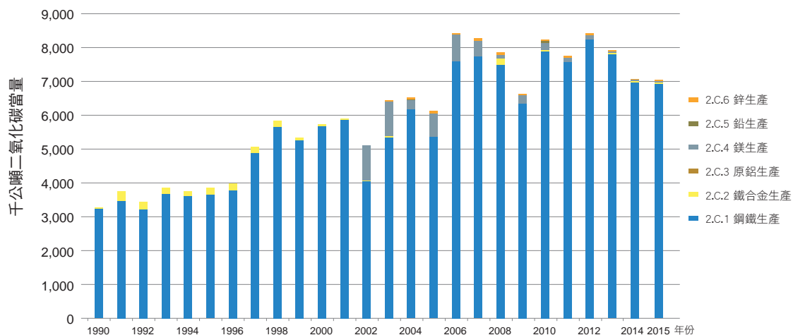
圖 4.4.1 臺灣 1990 至 2015 年金屬製程排放量趨勢
