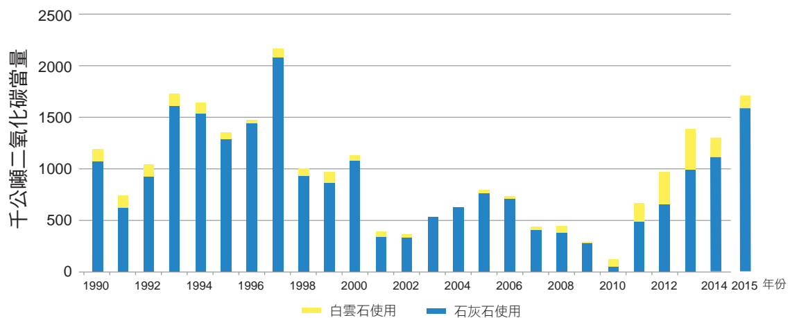
圖 4.2.8 臺灣 1990 至 2015 年石灰石與白雲石使用排放量趨勢
