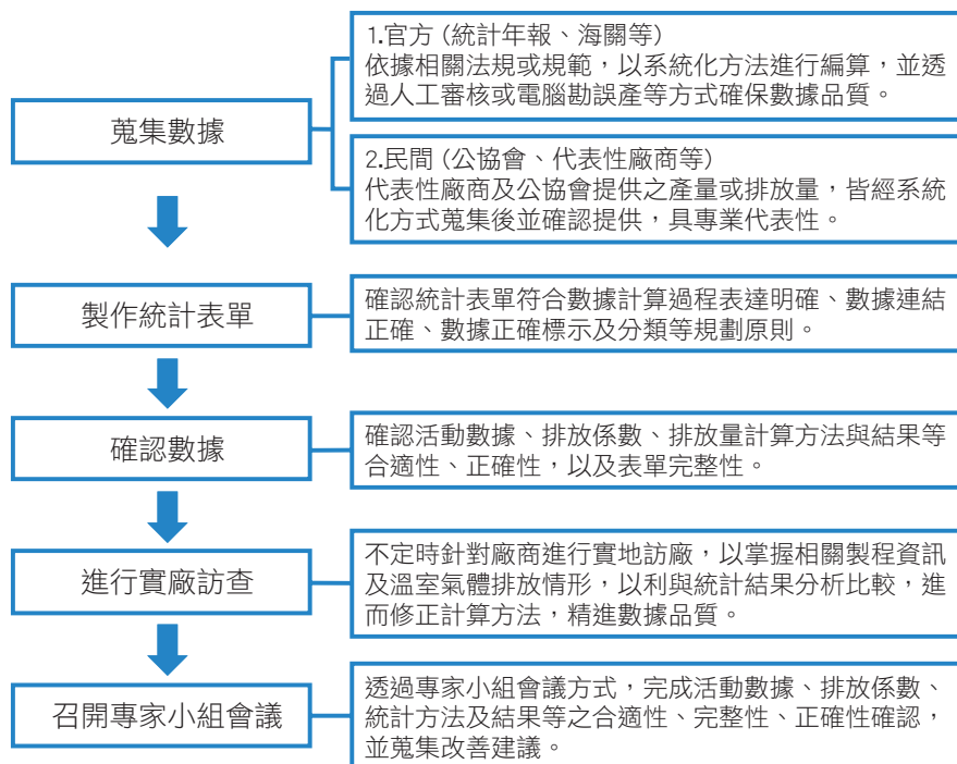
圖 4.3.3 工業製程及產品使用部門溫室氣體排放統計 QA/QC 流程（活動數據 - 官方數據、公協會及廠商來源）
