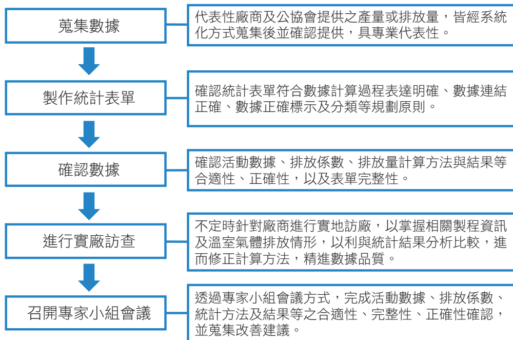
圖 4.2.3 工業製程及產品使用部門溫室氣體排放統計 QA/QC 流程（活動數據 - 廠商、公會及協會來源）
