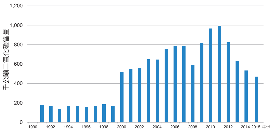
圖 4.3.4 臺灣 1990 至 2015 年己內醯胺生產排放量趨勢
