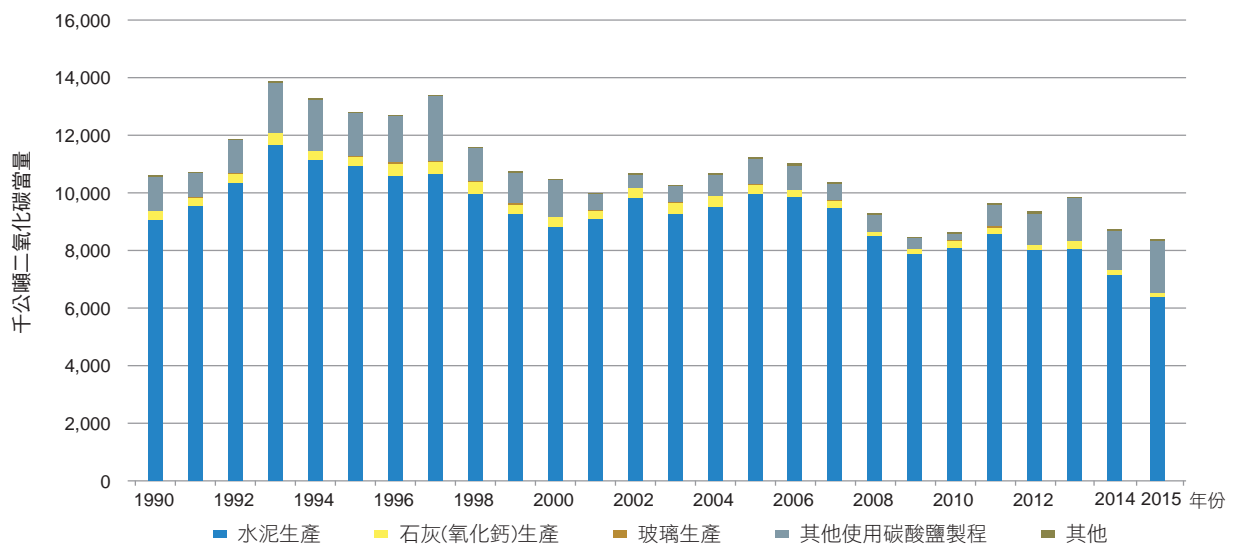
圖 4.2.1 臺灣 1990 至 2015 年礦業（非金屬製程）排放量趨勢
