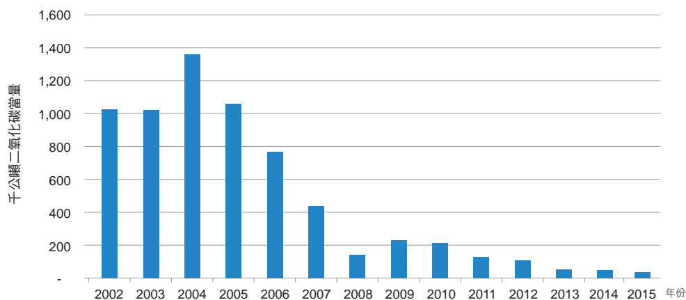
圖 4.4.5 臺灣 2002 至 2015 年鎂生產排放量趨勢
