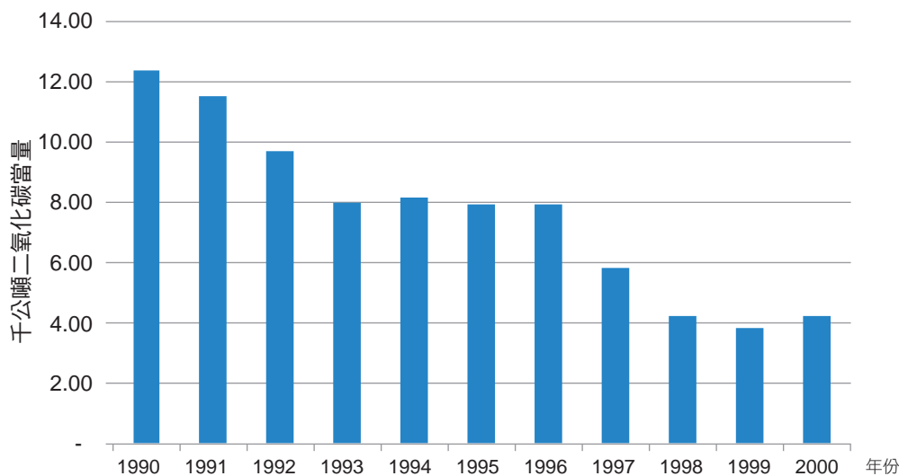
圖 4.3.7 臺灣 1990 至 2000 年純鹼生產排放量
