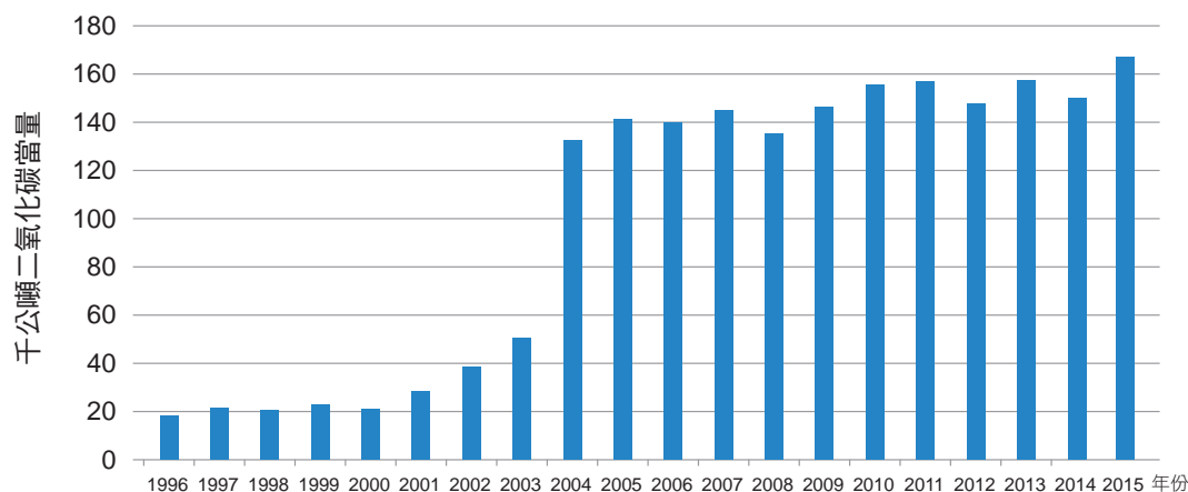
圖 4.3.11 臺灣 1996 至 2015 年環氧乙烷生產排放量趨勢
