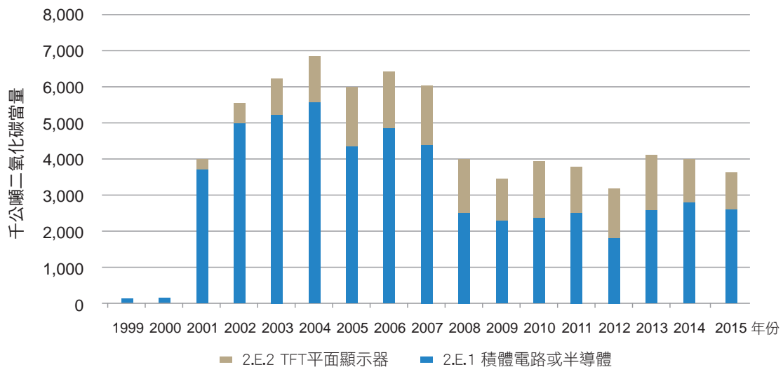
圖 4.6.1 臺灣 1999 至 2015 年電子工業排放量趨勢
