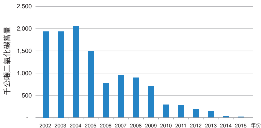
圖 4.8.1 臺灣 2002 至 2015 年高壓斷路器及其他開關絕緣氣體排放量趨勢
