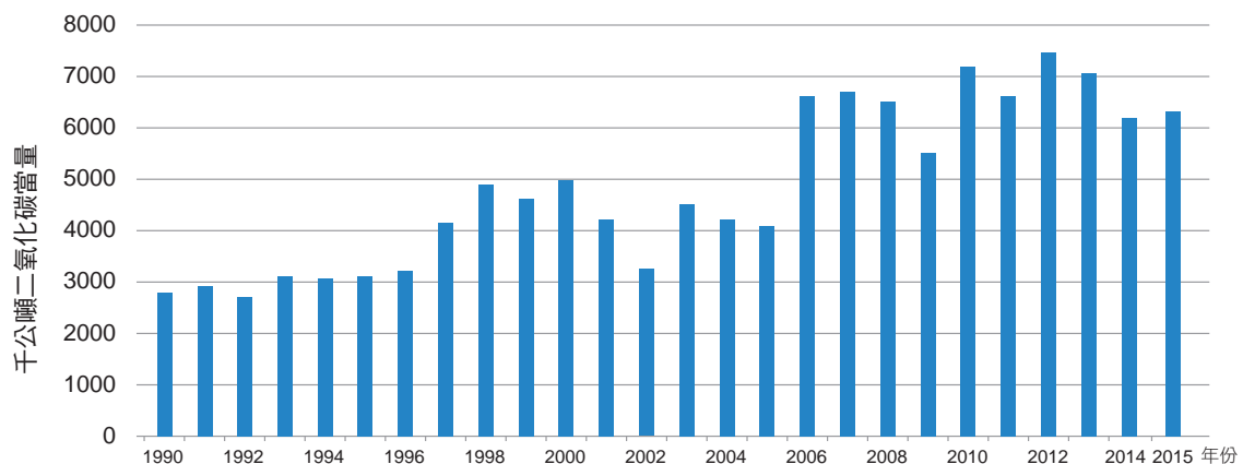
圖 4.4.2 臺灣 1990 至 2015 年高爐鋼胚生產排放量趨勢
