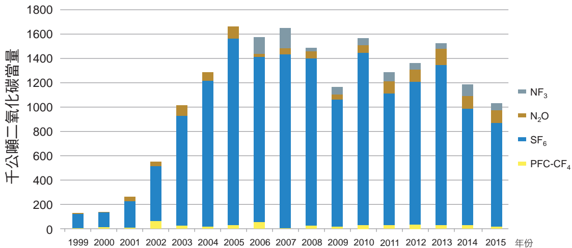
圖 4.6.4 臺灣 1999 至 2015 年 TFT 平面顯示器排放量趨勢
