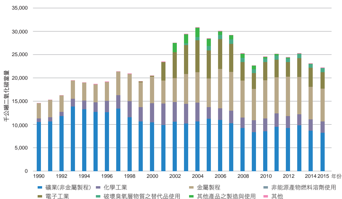
圖 4.1.3 臺灣 1990 至 2015 年工業製程及產品使用部門排放量趨勢
