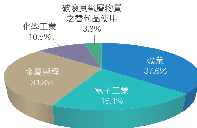
圖 4.1.2 臺灣 2015 年工業製程及產品使用部門溫室氣體排放占比
