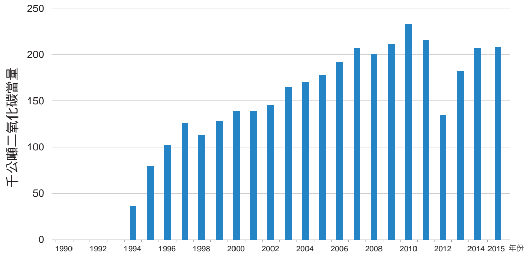
圖 4.3.6 臺灣 1990 至 2015 年二氧化碳生產排放量趨勢
