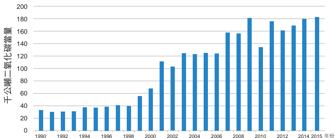
圖 4.3.9 臺灣 1990 至 2015 年乙烯生產排放量趨勢
