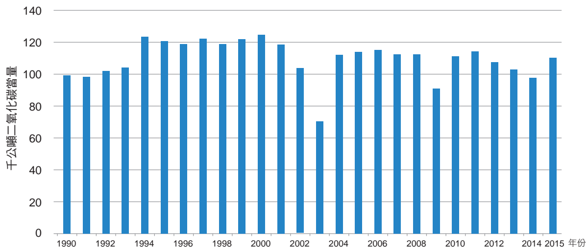
圖 4.2.7 臺灣 1990 至 2015 年純鹼使用排放量趨勢
