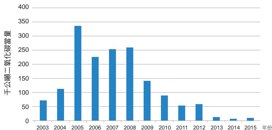
圖 4.7.3 臺灣 2003 至 2015 年滅火劑使用排放量趨勢
