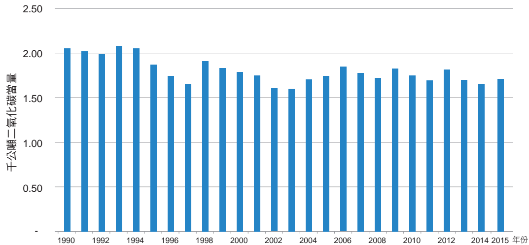
圖 4.9.1 臺灣 1990 至 2015 年啤酒生產排放量趨勢
