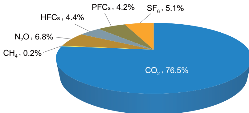
圖 4.1.1 臺灣 2015 年工業製程及產品使用部門溫室氣體種類排放占比
