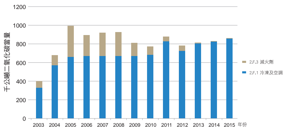
圖 4.7.1 臺灣 2003 至 2015 年破壞臭氧層物質之替代品使用排放量趨勢
