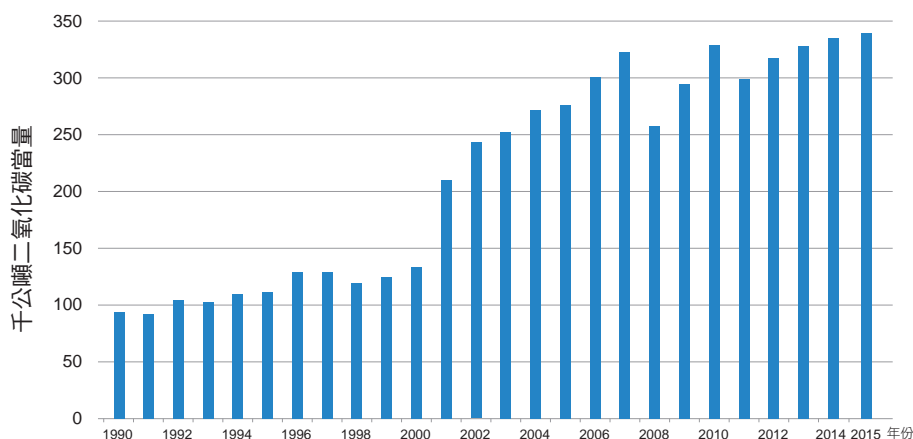
圖 4.3.12 臺灣 1990 至 2015 年丙烯腈生產排放量趨勢
