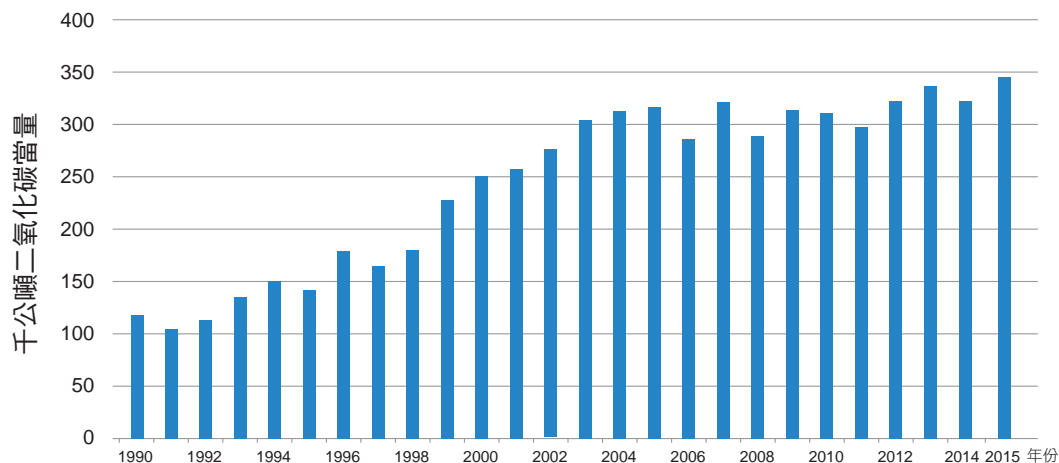
圖 4.3.10 臺灣 1990 至 2015 年氯乙烯生產排放量趨勢
