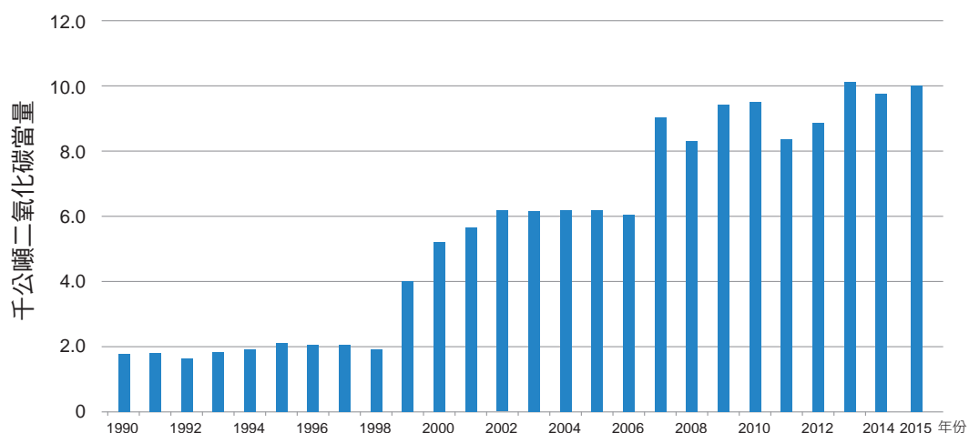
圖 4.3.15 臺灣 1990 至 2015 年苯乙烯生產排放量趨勢
