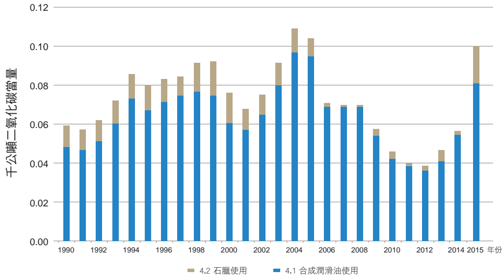
圖 4.5.1 臺灣 1990 至 2015 年非能源產物燃料溶劑使用排放量趨勢
