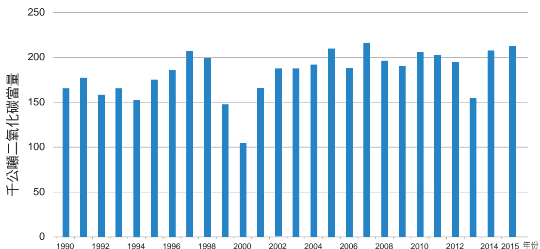
圖 4.3.2 臺灣 1990 至 2015 年硝酸生產排放量趨勢
