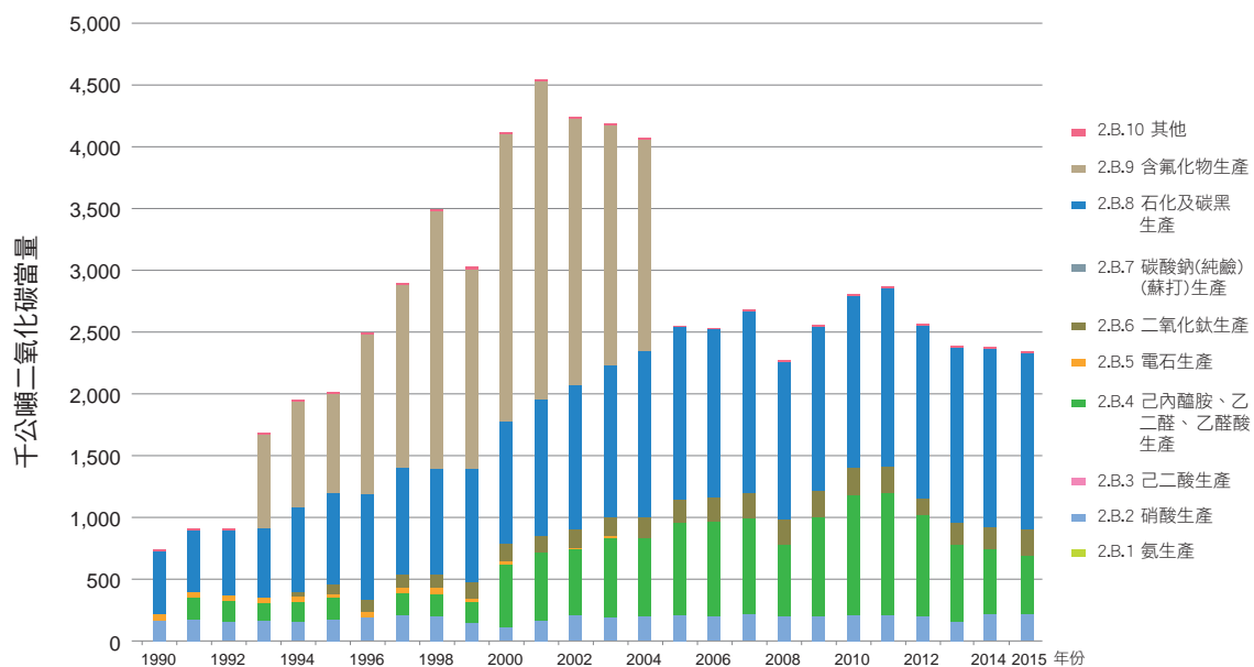
圖 4.3.1 臺灣 1990 至 2015 年化學工業排放量趨勢
