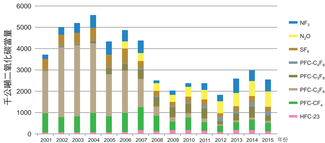
圖 4.6.2 臺灣 2001 至 2015 年積體電路或半導體排放量趨勢
