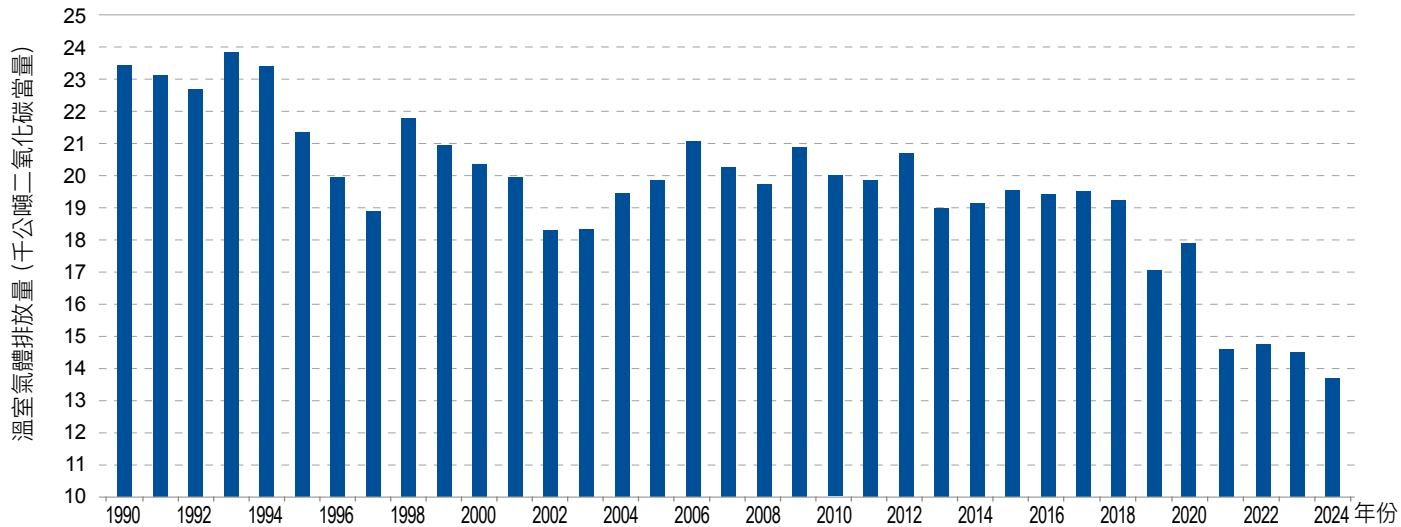
圖 4.9.2 1990 年至 2024 年啤酒生產製程排放量趨勢
