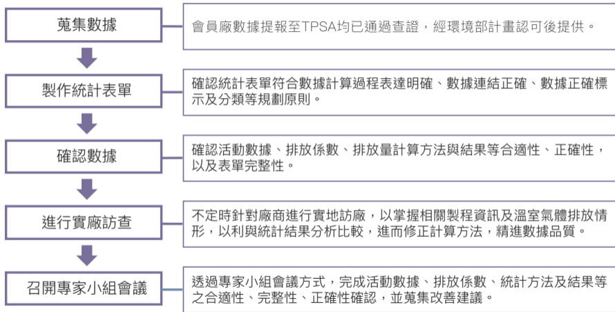
圖 4.6.5 TFT 平面顯示器製程排放統計 QA/QC 流程
