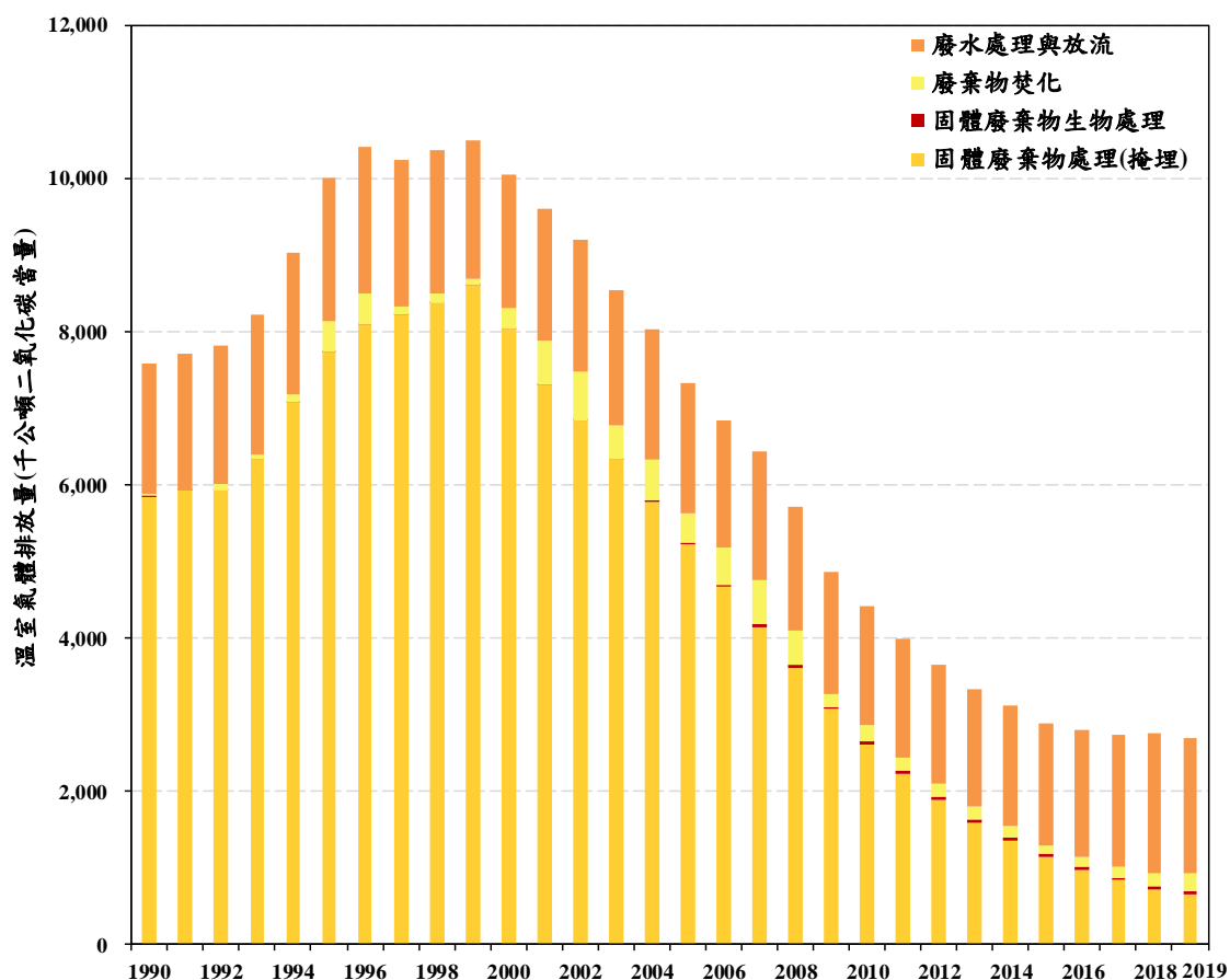
圖 7.1.1 臺灣 1990 年至 2019 年廢棄物部門各類排放源溫室氣體排放量趨勢
