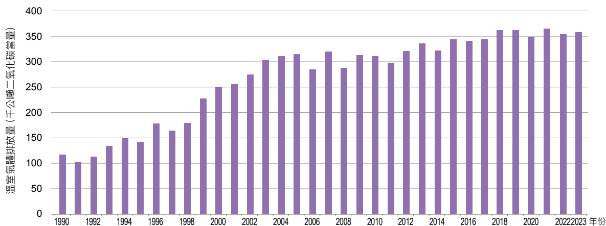
圖 4.3.9 1990 年至 2023 年氯乙烷生產製程排放量趨勢
