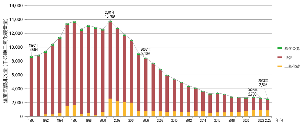
圖 7.1.4 1990 年至 2023 年廢棄物部門各類溫室氣體排放量趨勢
