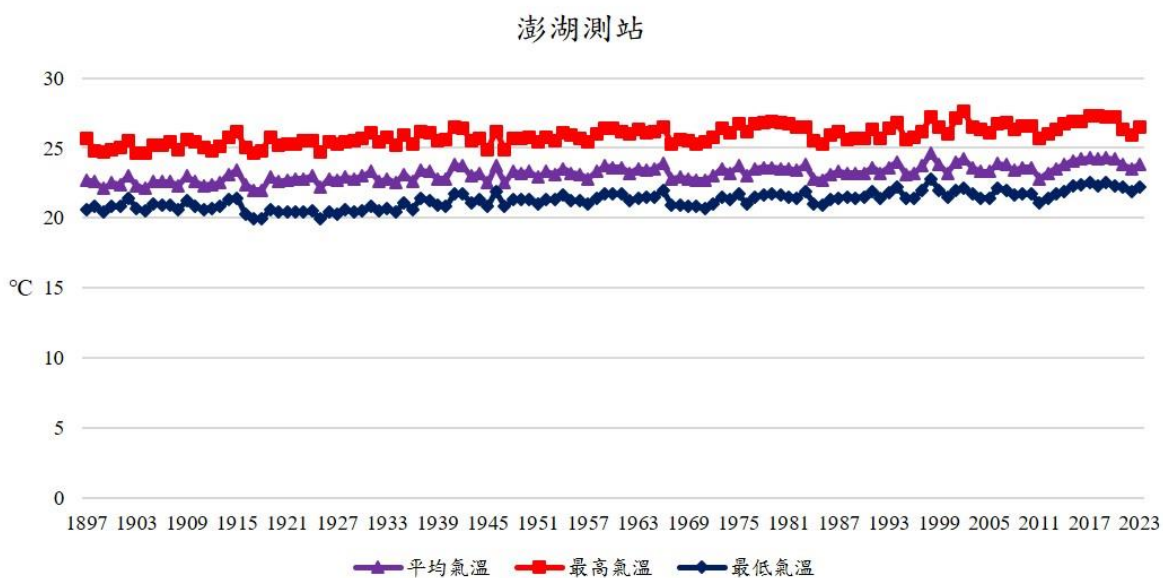
圖 2.16 澎湖測站歷年平均氣溫
