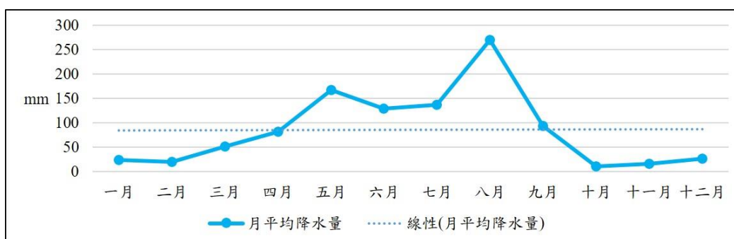
資料來源：CODis 氣候資料服務系統；交通部中央氣象署(2013-2023)；本計畫彙整 圖 2.3 澎湖縣近年(2013年~2023年)月平均降雨趨勢圖
