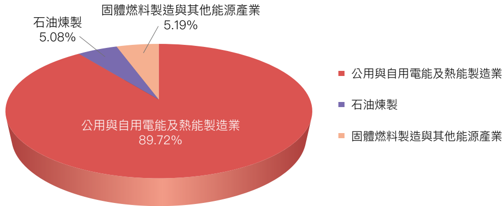
圖 3.2.18 2024 年能源產業各排放源燃料燃燒二氧化碳排放占比
