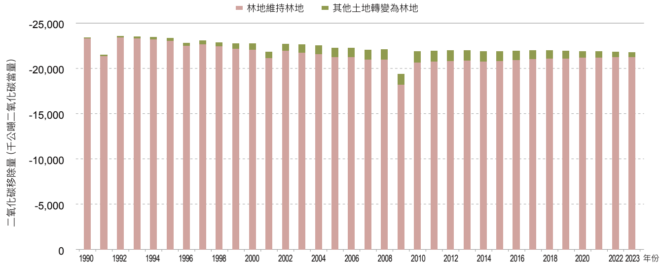
圖 6.2.1 1990 年至 2023 年林地碳移除量變化趨勢
