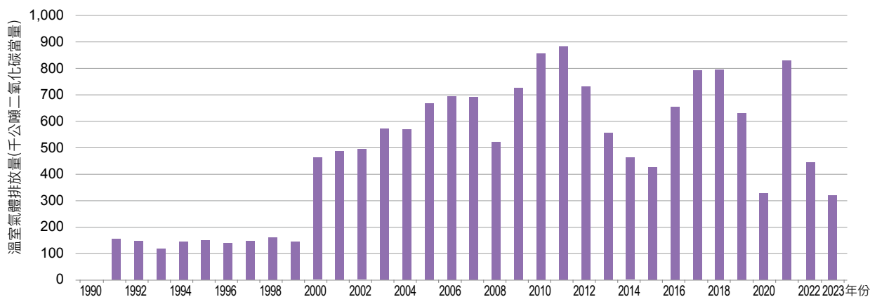
圖 4.3.3 1990 年至 2023 年己內醯胺生產製程排放量趨勢
