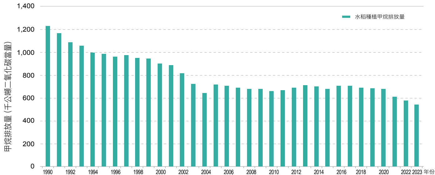
圖 5.4.1 1990 年至 2023 年水稻種植甲烷排放量
