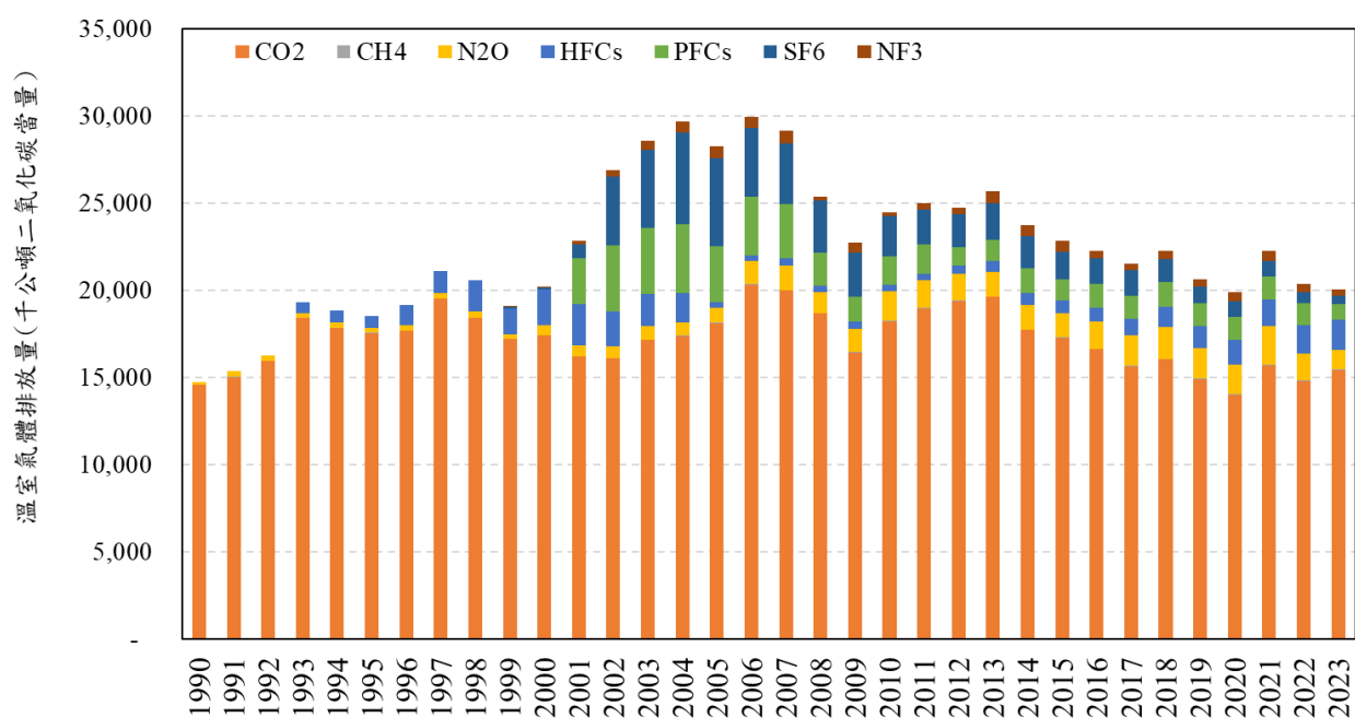
圖 4.1.4 1990 年至 2023 年工業製程及產品使用部門排放量趨勢（依氣體）
