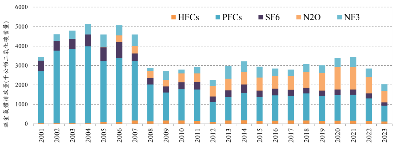
圖 4.6.2 2001 年至 2023 年積體電路及半導體製程排放量趨勢
