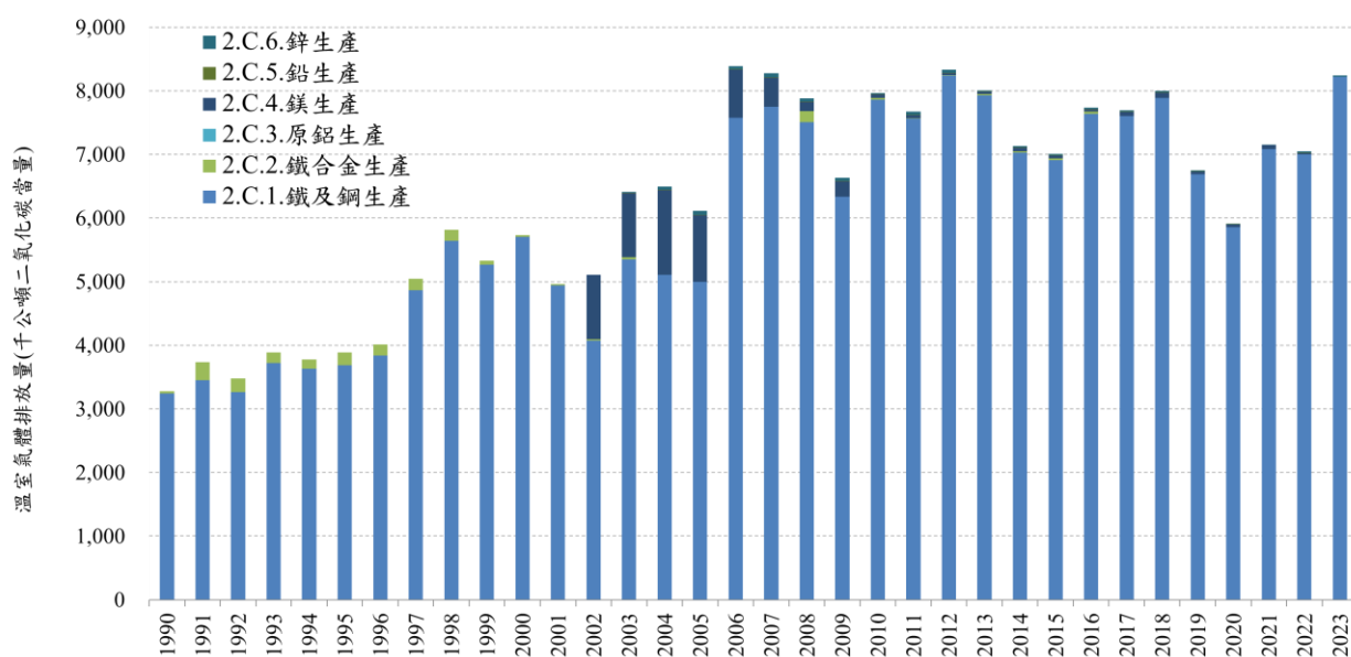
圖 4.4.1 1990 年至 2023 年金屬工業排放量趨勢
