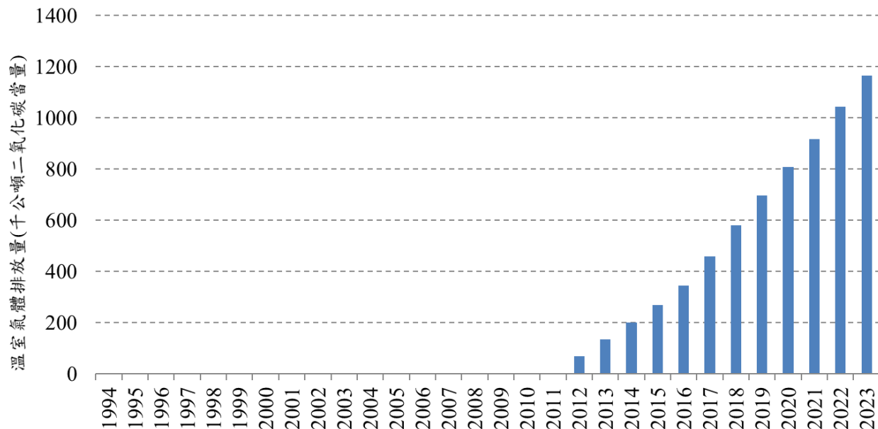
圖 4.7.4 1994 年至 2023 年固定式空調之 HFCs 排放量趨勢
