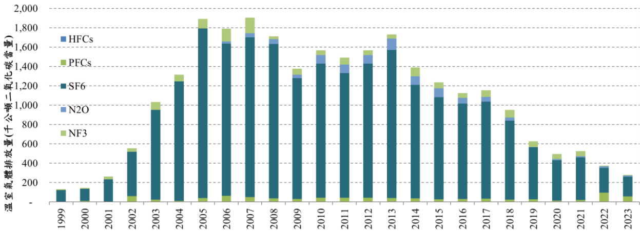
圖 4.6.3 1999 年至 2023 年 TFT 平面顯示器製程排放量趨勢
