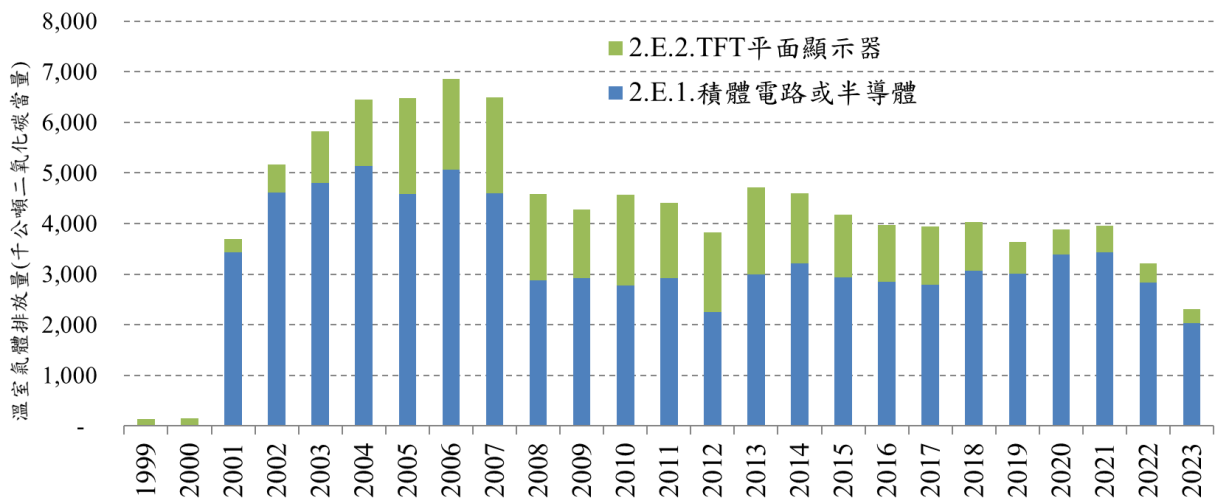
圖 4.6.1 1999 年至 2023 年電子工業製程排放量趨勢
