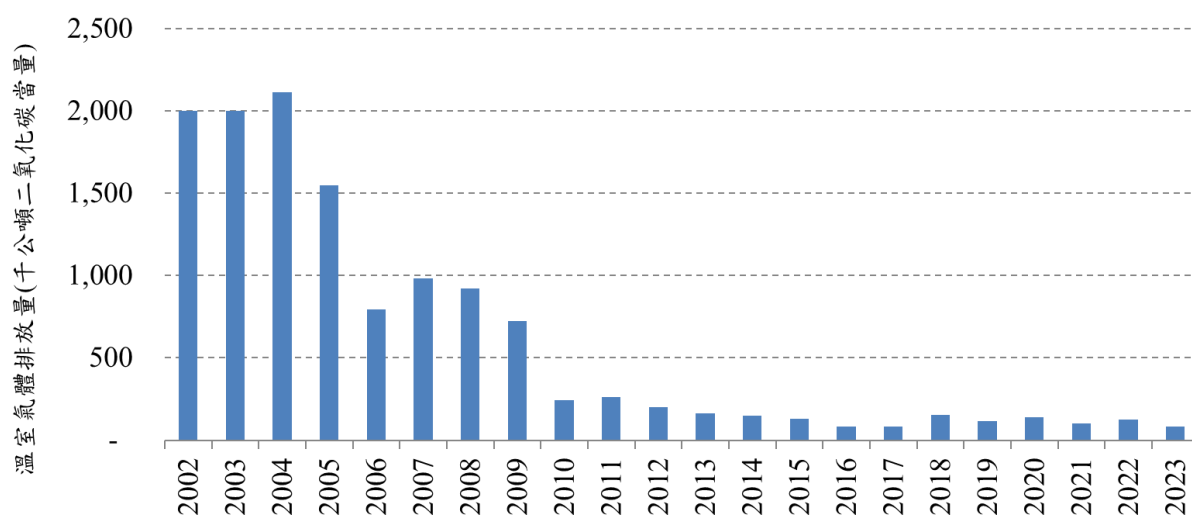
圖 4.8.1 2002 至 2023 年電力設備中之六氟化硫排放趨勢
