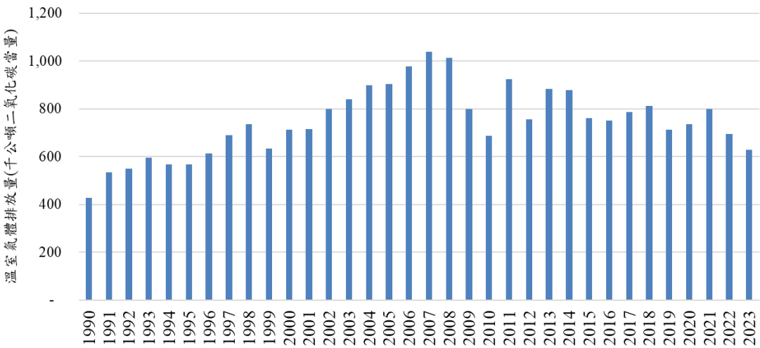
圖 4.4.3 1990 年至 2023 年電弧爐鋼胚生產製程排放量趨勢
