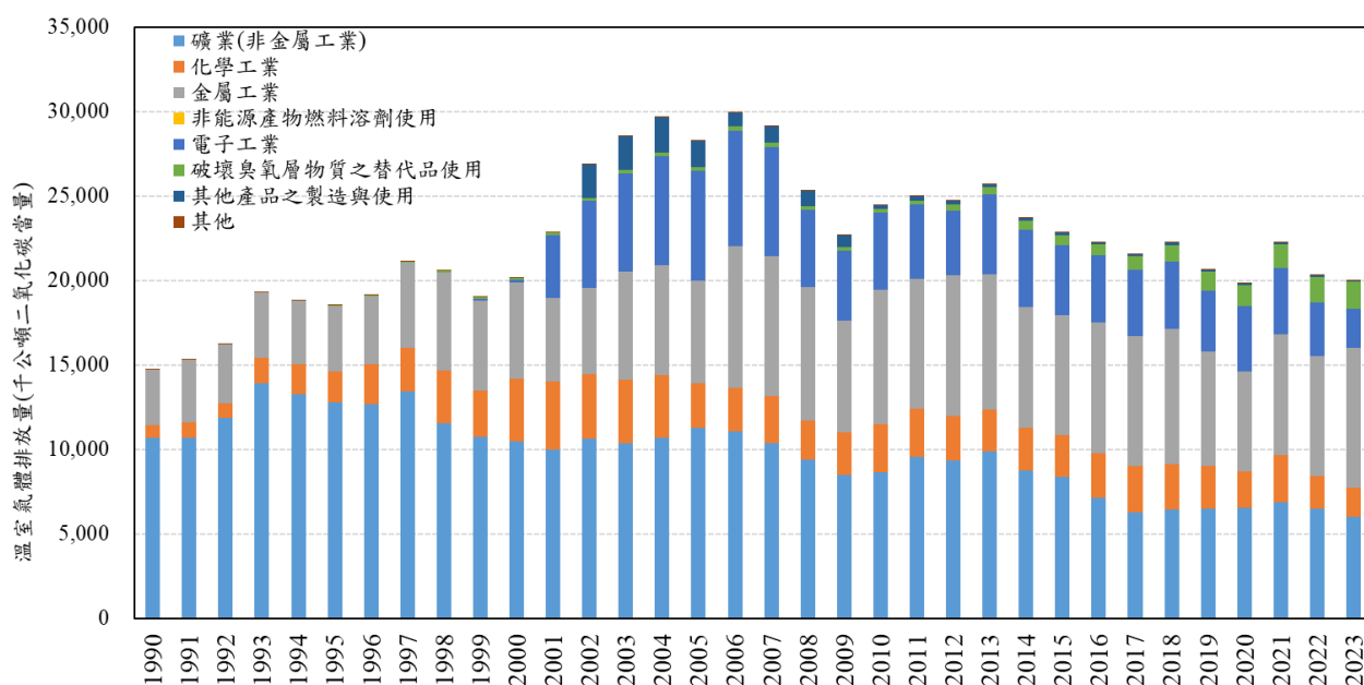
圖 4.1.3 1990 年至 2023 年工業製程及產品使用部門排放量趨勢（依類別）
