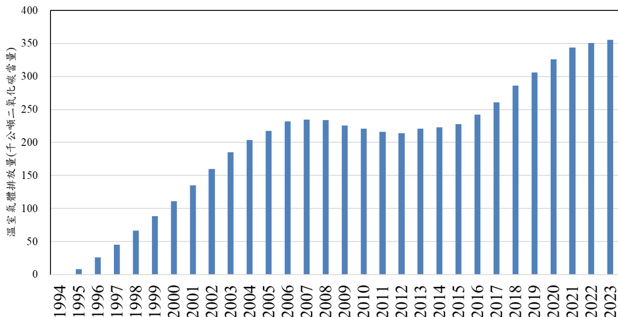
圖 4.7.3 1994 年至 2023 年車用空調之 HFCs 排放量趨勢
