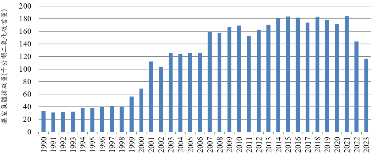
圖 4.3.8 1990 年至 2023 年乙烯生產製程排放量趨勢
